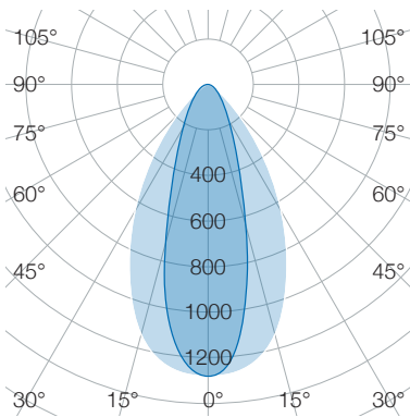
ClickLUX 2.0 SL 25° x 60°
