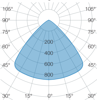
ClickLUX 2.0 SL 90°
