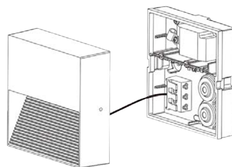
EASYbase für einfache Montage
