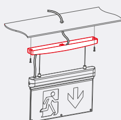
Deckenmontage, abgehängt
