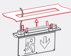
Deckenmontage, mit Einbaurahmen
