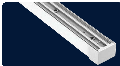
Zwei Kabeleingänge ermöglichen flexible Montage bei vorhandenen Kabelauslässen
