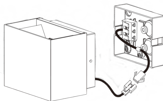
EASYbase für einfache Montage
