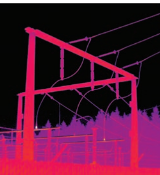
Überhitzte Bereiche an elektrischen Anlagen
