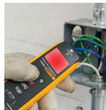
Schnelle Überprüfung auf anliegende Spannung ohne Berührung eines spannungsführenden Leiters
