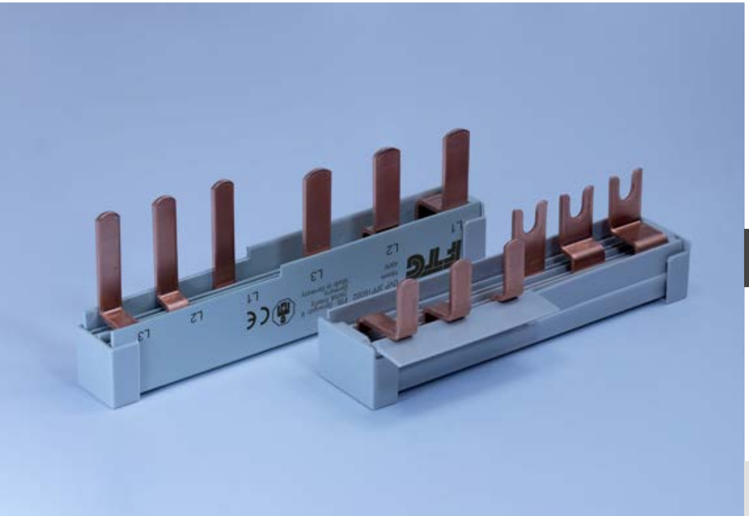
Phasenschielen für Überspannungsableiter | Busbars for Overvoltage Protection Devices | Peignes pour parasurtensions
