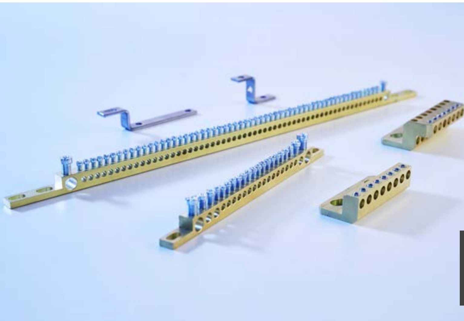
Null- und Schutzleiterklemmen | Neutral and earthing terminals | Barres de neutre et terre
