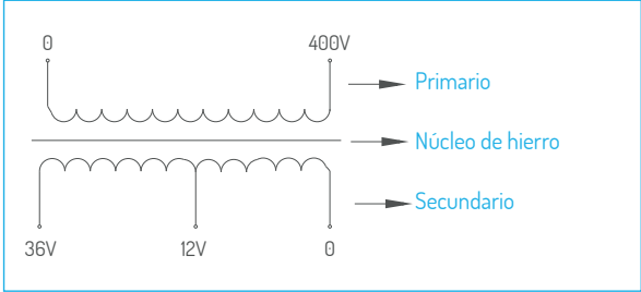
1 ENTRADA - 2 SALIDAS
