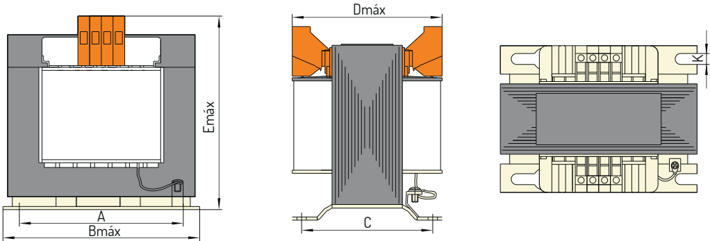
Dimensiones (mm)
