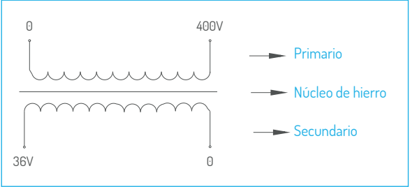
1 ENTRADA - 1 SALIDA
