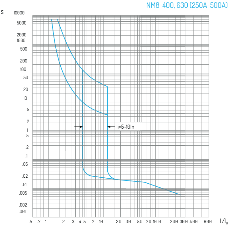
CURVAS DE DISPARO / Modelos NM8-400 / NM8-630 (T3)
