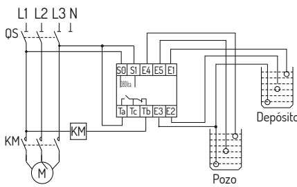
NJYW1-BL2 (Modo pozo y depósito)
