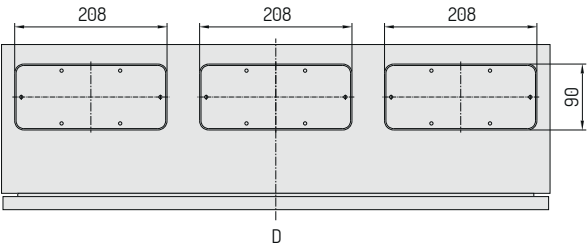
ENTRADA DE CABLES / Tipo D
