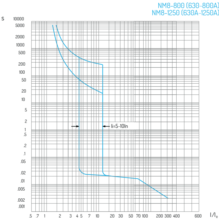
CURVAS DE DISPARO / Modelos NM8-800 / NM8-1250 (T4)
