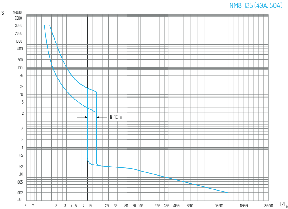
CURVAS DE DISPARO / Modelo NM8-125 (T1)
