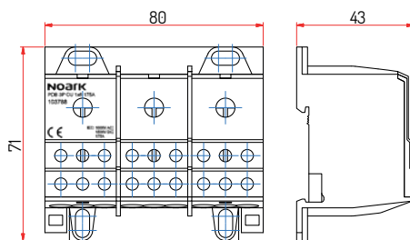
PDB 3P CU 1x6 175A
