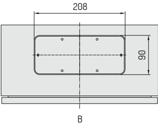
ENTRADA DE CABLES / Tipo B
