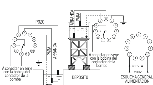
CNT1: Control de pozo y depósito
