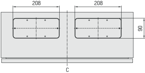
ENTRADA DE CABLES / Tipo D
