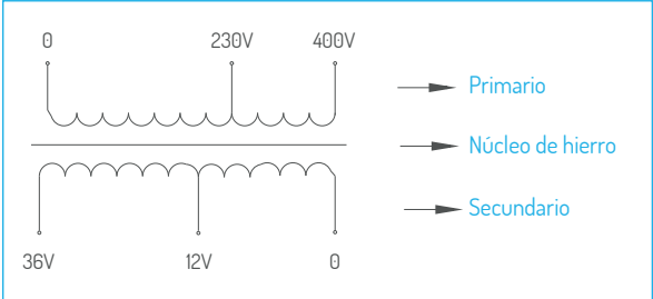
2 ENTRADAS - 2 SALIDAS
