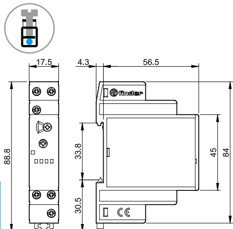
80.41T Borne de jaula
