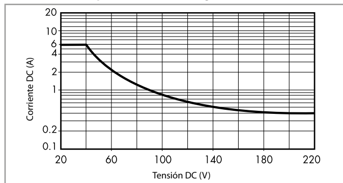
H 7S16* - Máximo poder de corte con cargas en DC - 7S.16
