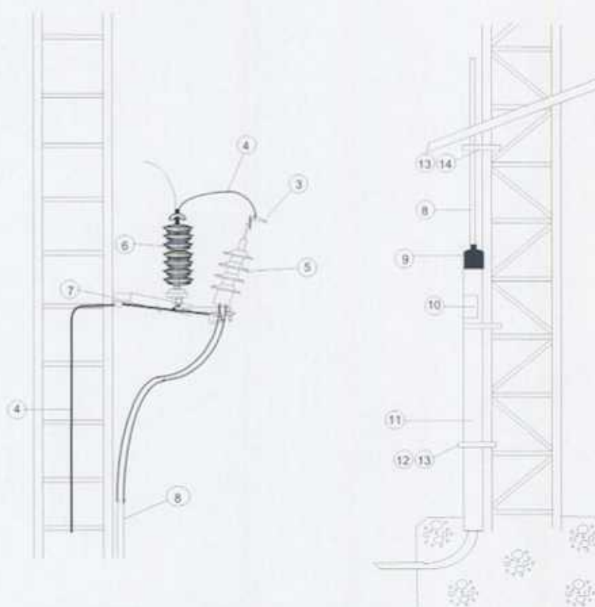
ENTRONQUE AÉREO SUBTERRÁNEO
