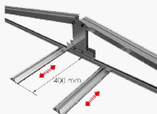
Fácil regulación del portalastré simplemente aflojando un tornillo (Ejemplo de portalastré descentrado).
