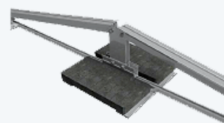
Ejemplo de instalación de 2 contrapesos de 1 de hasta 200 mm de ancho repartidos sobre portalastré.
