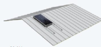
01.1H Disposición de los módulos en horizontal
