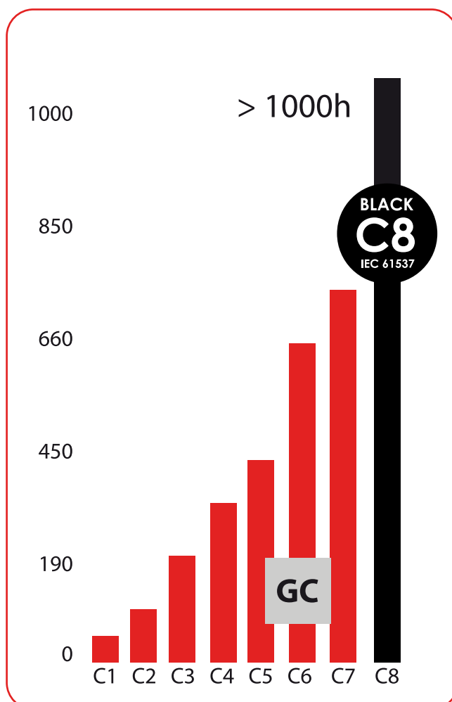
Duración (h) ensayo Camara niebla salina, según ASTM-B117 Duração (h) Teste Camara de nuvem salina, conforme ASTM-B117
