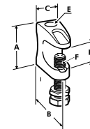
Dimensiones (mm)
