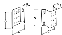
Dimensiones (mm)
