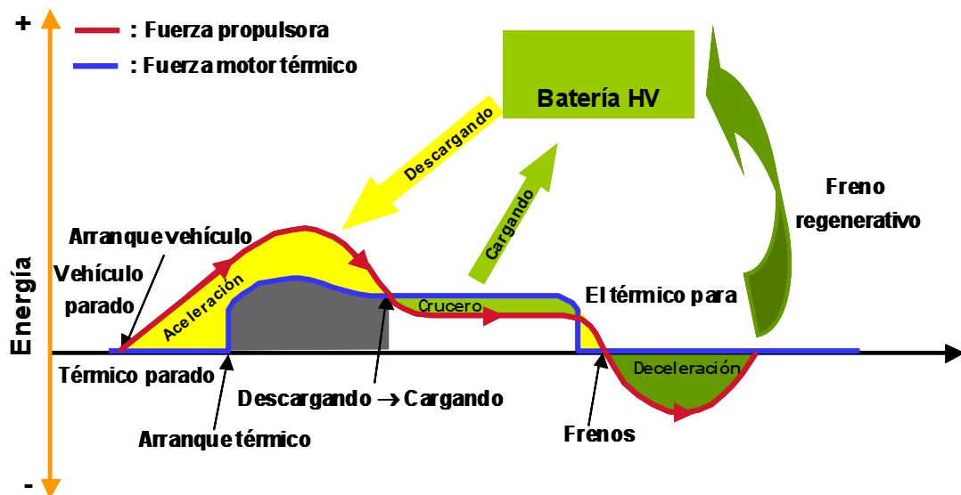
Figura 4.2. Esquema de funcionamiento de un sistema de hibridación.
