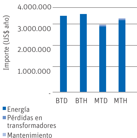
GRÁFICO 7.1 Comparación de costos por tarifa
