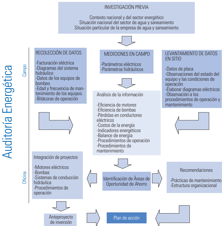
GRÁFICO 2.1 Metodología para realizar una auditoría energética
