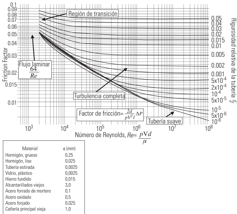
GRÁFICO 6.11 Diagrama de Moody
