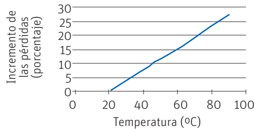
GRÁFICO 6.4 Pérdidas en transformadores en función de la temperatura
