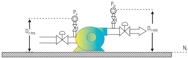
GRÁFICO 5.7 Medición de niveles en caso de contar con manómetros en succión y descargas.
