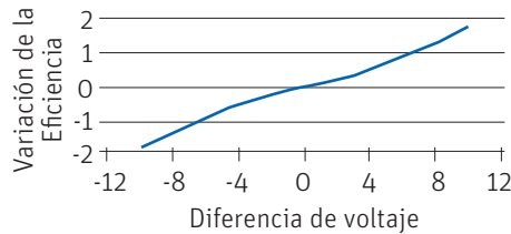
GRÁFICO 6.7 Puntos de eficiencia a depreciar en función de la diferencia de voltaje con respecto a la nominal en un motor eléctrico
