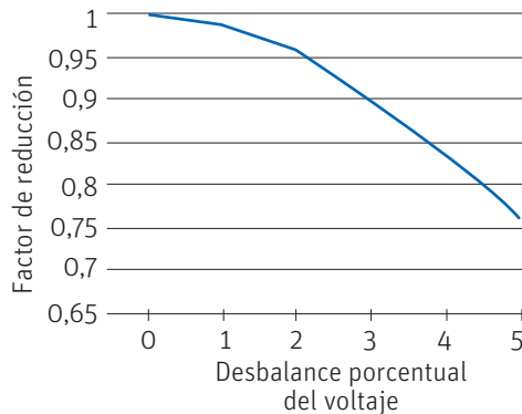
GRÁFICO 6.8 Reducción porcentual de la eficiencia de un motor eléctrico en función del desbalance de voltaje
