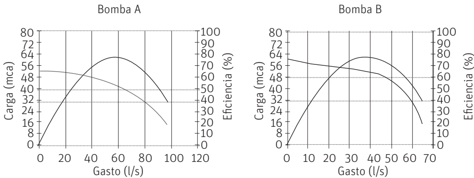
GRÁFICO 7.2 Curva típica de dos equipos de bombeo con curvas H-Q diferentes
