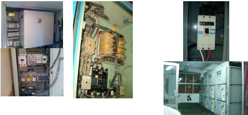
FOTOGRAFÍA 6.2 Componentes típicos del sistema electromotriz de un sistema de bombeo
