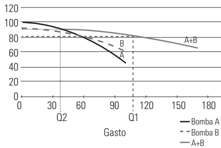
GRÁFICO 6.13 Características de carga-capacidad de bombas centrífugas operadas en paralelo
