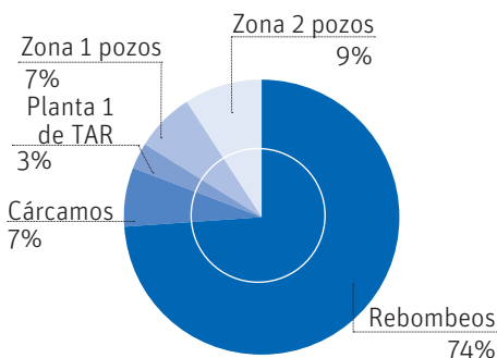
GRÁFICO 6.2 Descripción gráfica del balance de energía del sistema
