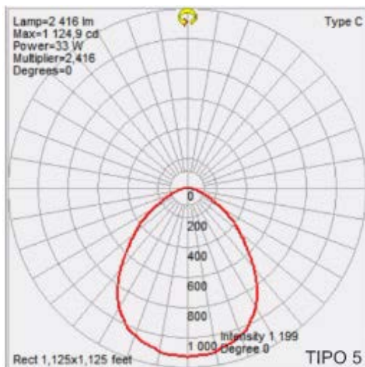
Figura 8.6. Distribución luminosa.
