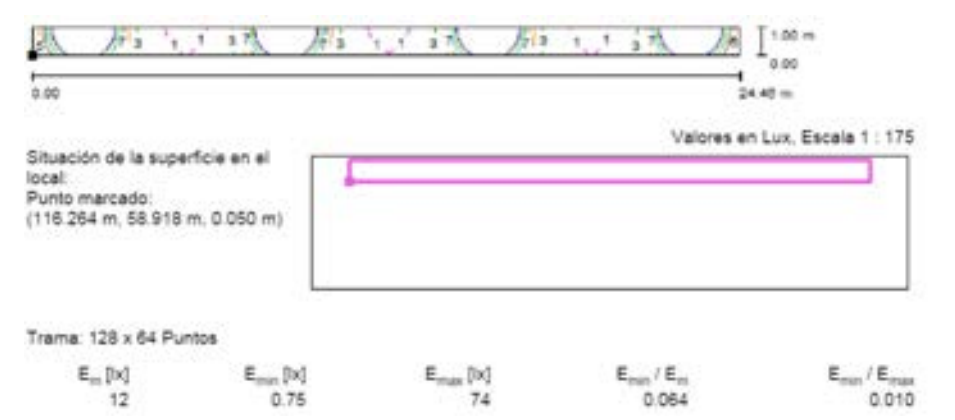
Figura 8.33. Luminancias ortogonales.
