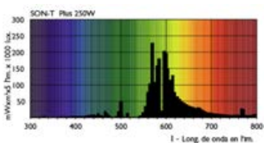
Figura 2.18. Espectro emisor de SON-T. Fuente: Philips.
