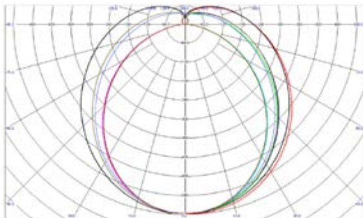
Figura 4.16. Distribución lumínica.
