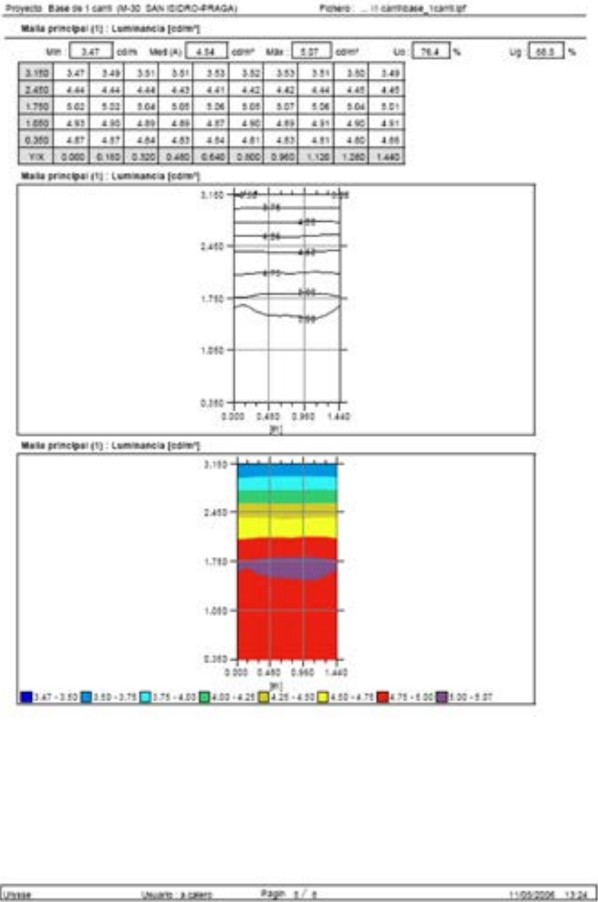
Figura 8.27. Iluminación zona de transición 3. (I).
