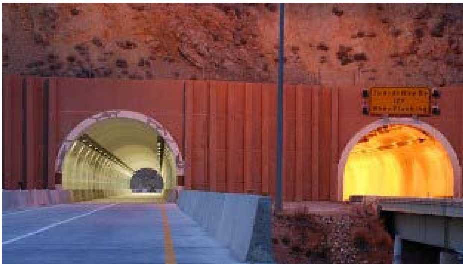
Figura 2.21. Comparativa boca de entrada y boca de salida.
