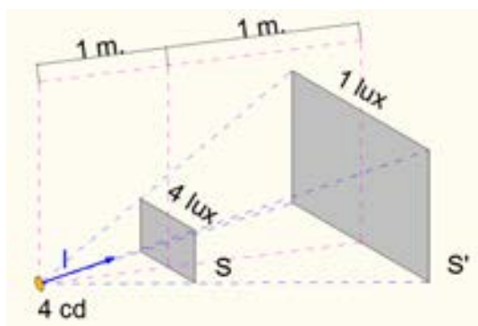
Figura 2.5. Definición de lux.
