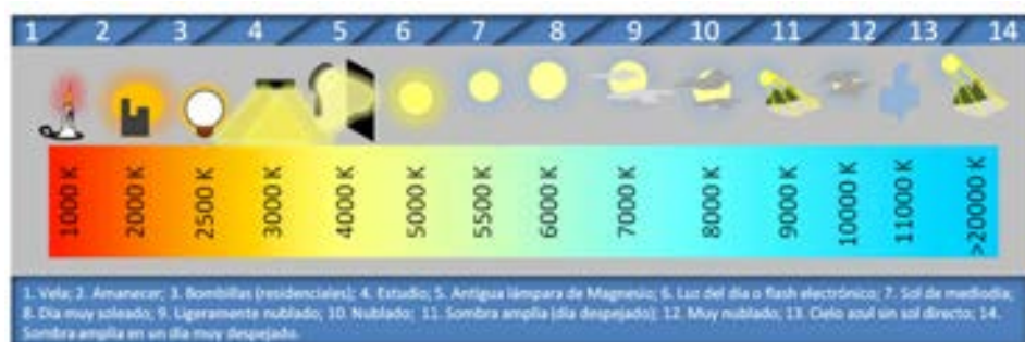
Figura 2.9. Temperatura del color.
