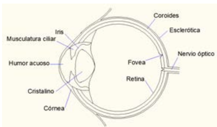
Figura 2.4. Esquema sobre la anatomía del ojo humano.
