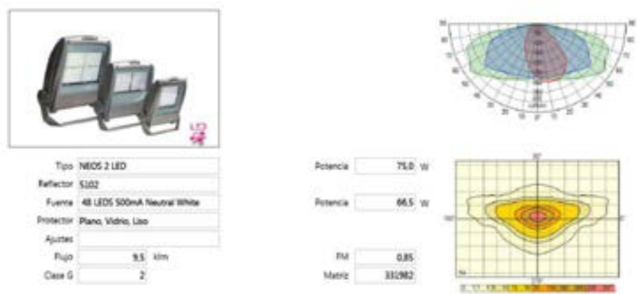
Figura 8.16. Esquemas lumínicos.
