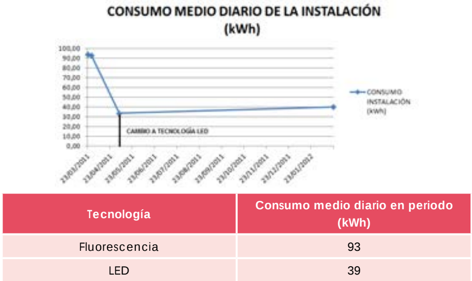
Figura 7.6. Consumos medios. Fuente: Madrid Calle 30.
