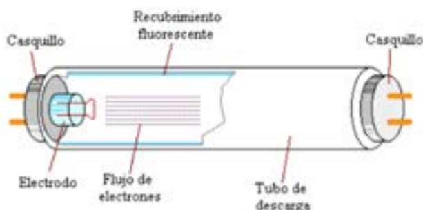
Figura 2.16. Esquema de un tubo fluorescente.
