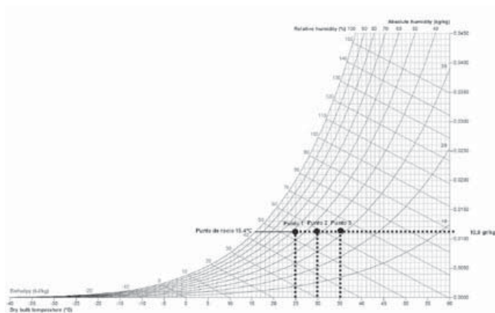
Figura 6.6. Representación de un sistema de control basado en la humedad absoluta
