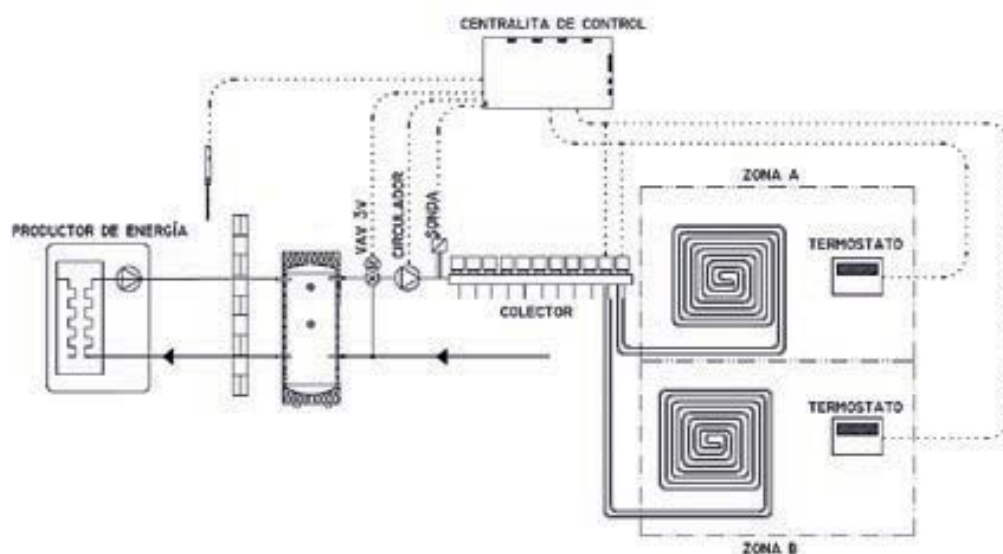
Figura 6.3. . Representación de termostatos de zona actuando sobre los cabezales y enviando información a la central de control para en función de la temperatura exterior actuar sobre la valvula de 3 vías o productor y modificar así la temperatura de agua.
