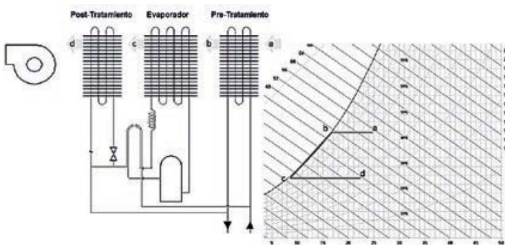
Figura 6.8. Esquemas del principio de funcionamiento de la deshumidificación isotérmica
