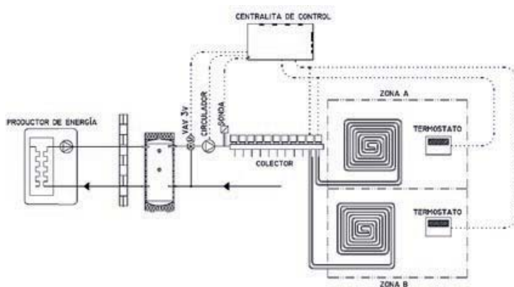
Figura 6.2. Representación de termostatos de zona actuando sobre los cabezales y enviando información a la central de control para gestión de la temperatura de agua a través de válvula de 3 vías.
