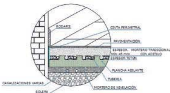
Figura 3.1a. Sección tipo de un suelo radiante
