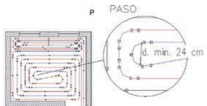
Figura 3.1b. Detalle circuito
