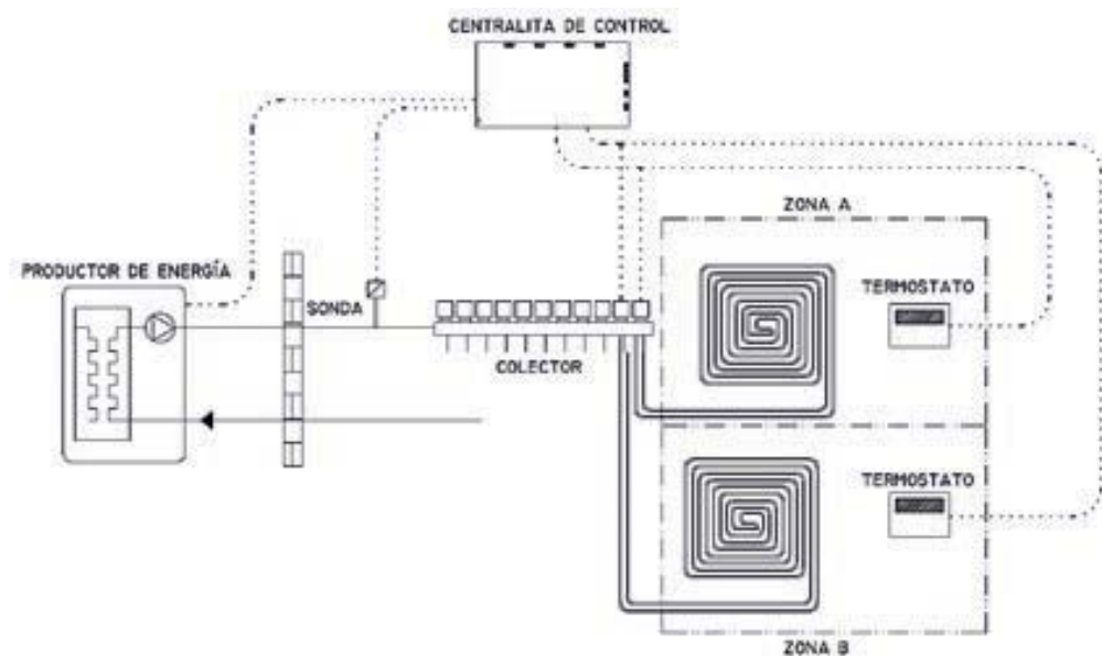
Figura 6.1. Representación de termostatos de zona actuando sobre los cabezales y enviando información a la central de control para gestión de la producción y temperatura de agua.
