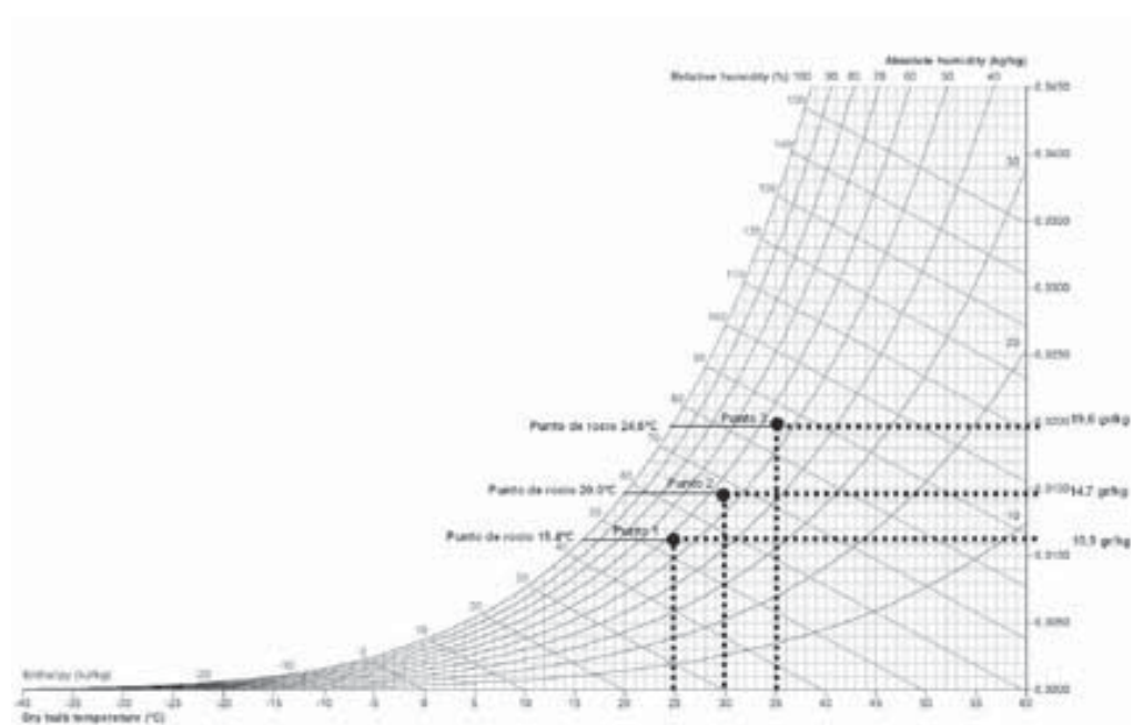
Figura 6.4. Representación de un sistema de control basado en la humedad relativa
