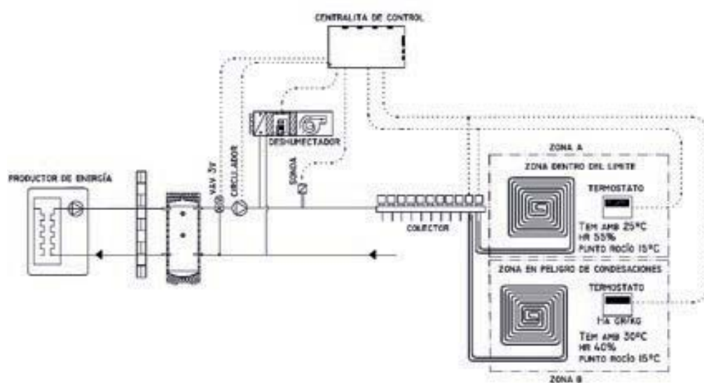
Figura 6.7. Representación de sistema de control por humedad absoluta con deshumectación, centralita de control y válvula de 3 vías controlada por la centralita en función del punto de rocío elaborado por cada termostato de control por humedad absoluta de cada zona.
