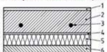
Sistemas tipo A: Tubo dentro del pavimento
