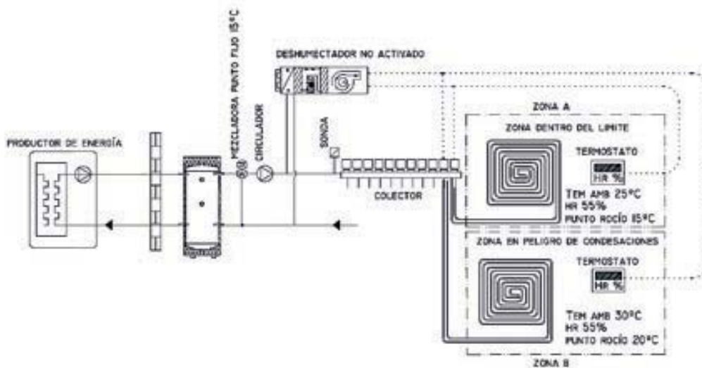
Figura 6.5. Representación de sistema de control por humedad relativa a deshumectación y mezcladora a punto fijo.
