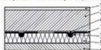
Sistemas tipo B: Tubo debajo del pavimento
