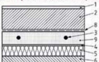
Sistemas tipo C: Tubo dentro del pavimento
