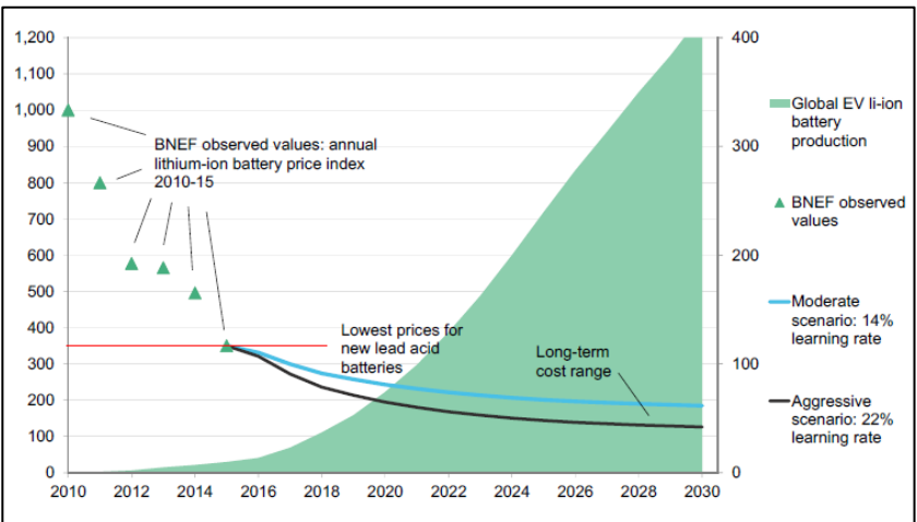
Precio de las baterías de ion Litio ($/kWh)
