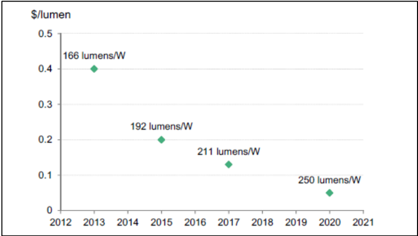
Eficacia y precio del LED ($/Lm)
