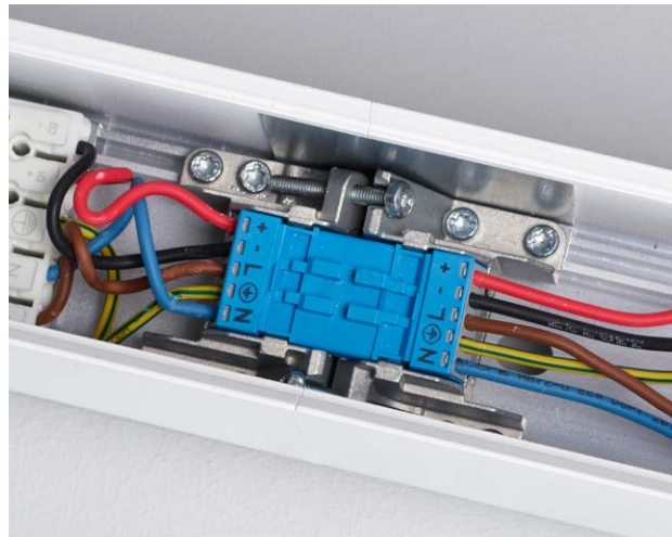
Conexión segura y firme
