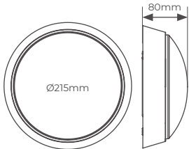
Productos suministrados con biseles blancos y negros intercambiables
