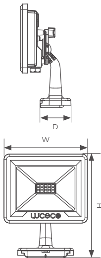
Soporte de instalación de 2 piezas
