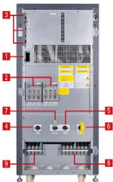
SLC-7,5÷200-CUBE3+
