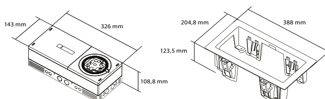
Kit d'encastrement ALTILED
