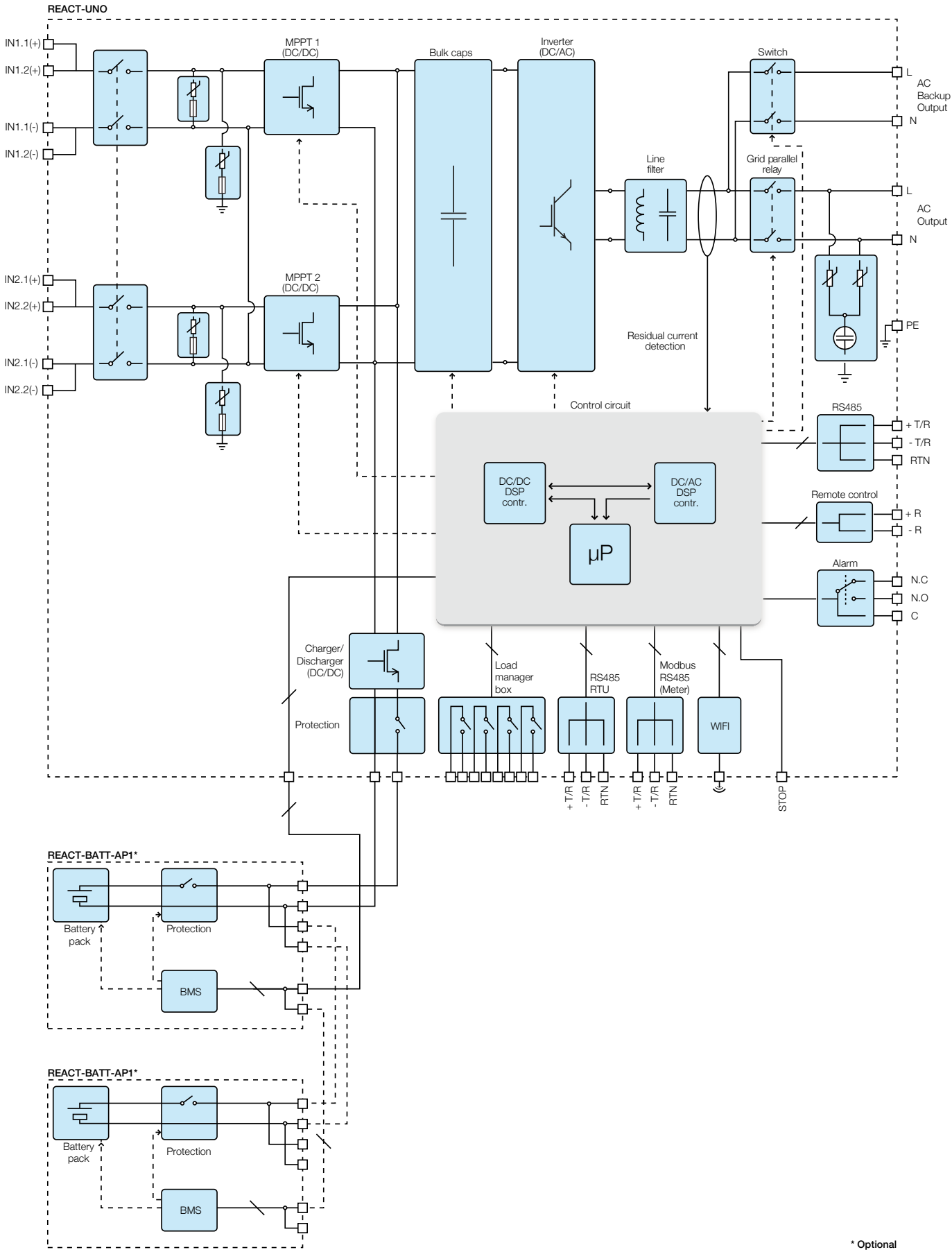
Diagramma a blocchi REACT-4.6
