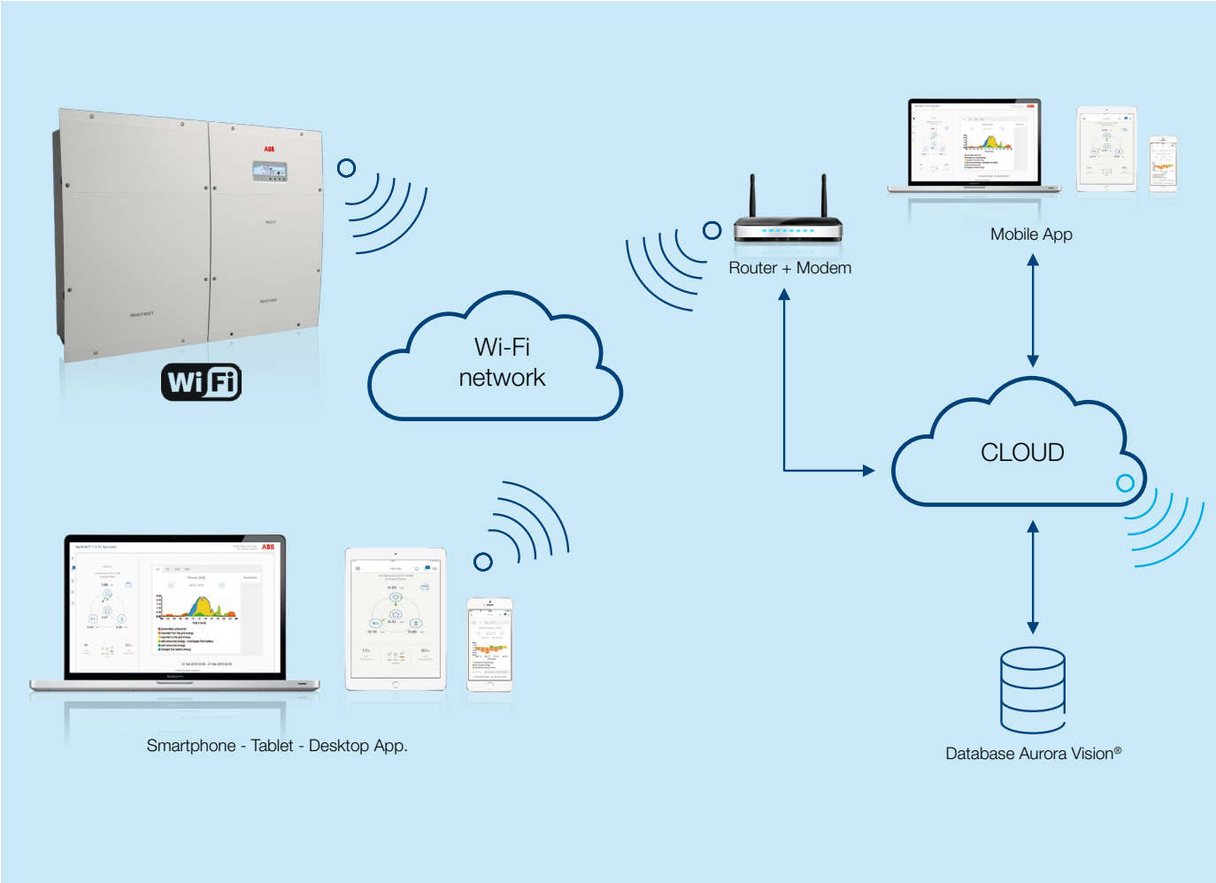
Diagramma a blocchi REACT-4.6
