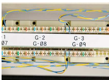
Etichette blocco a incastro
