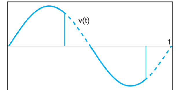
Trailing edge dimming
