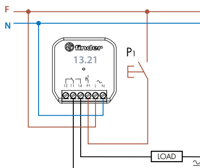
Collegamento con pulsante su fase
