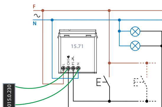
Dimmer 15.71.8.230.B20x
