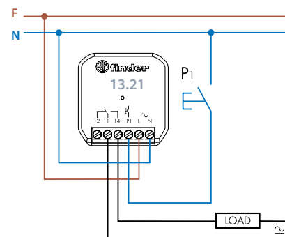
Collegamento con pulsante su neutro
