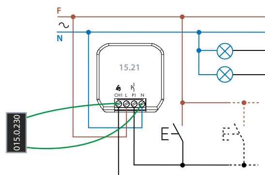
Dimmer 15.21.8.230.B300
