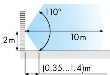
Area di rilevamento (vista laterale e in pianta)
