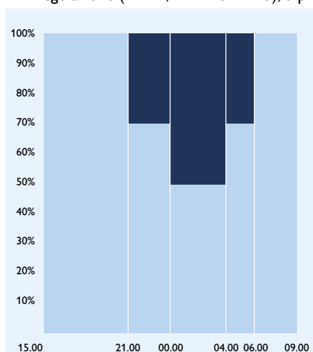
Programma standard DDF2, per un risparmio energetico fino al 32% rispetto alla versione senza regolazione del flusso
