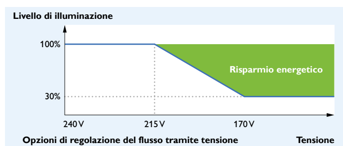
Programma standard DDF2, per un risparmio energetico fino al 32% rispetto alla versione senza regolazione del flusso
