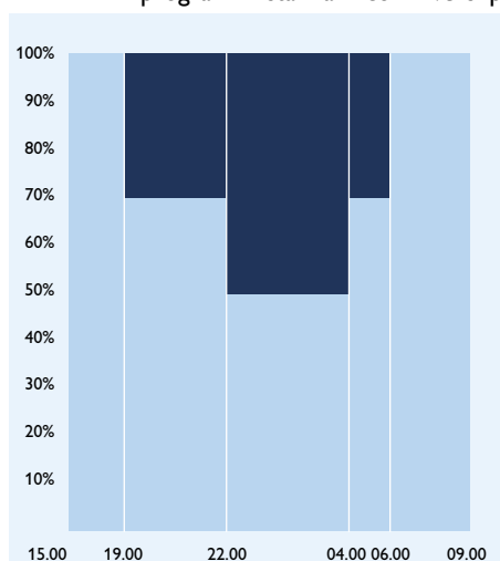
Programma standard DDF1, per un risparmio energetico fino al 40% rispetto alla versione senza regolazione del flusso
