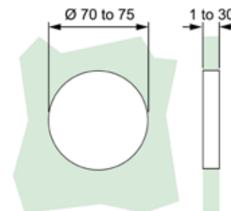
Dimensioni per l'incasso
