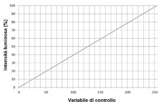
Figura 23. – Curva di dimming Lineare
