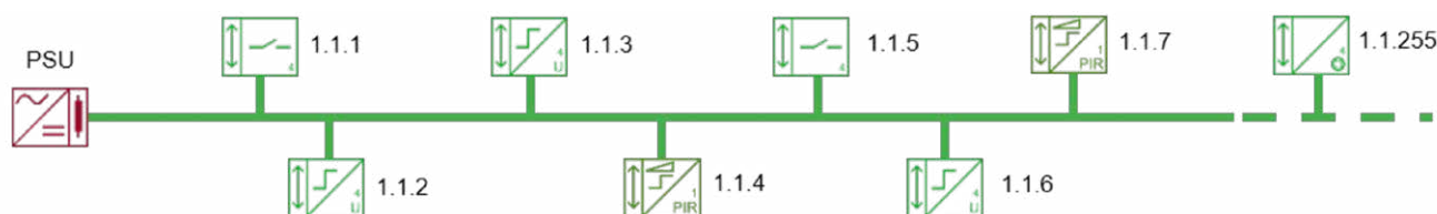
Figura 13. – Linea KNX TP1-256
