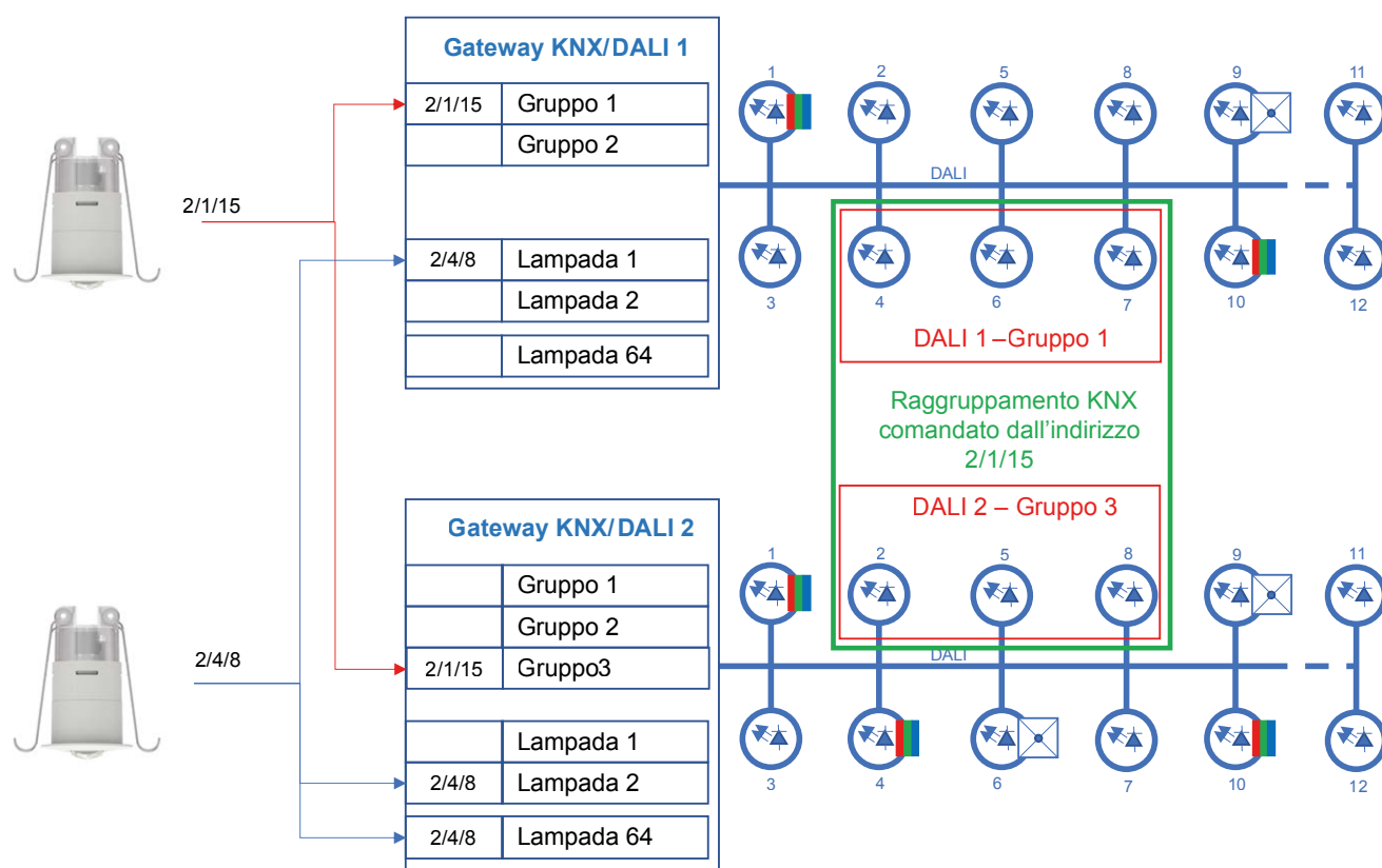
Figura 49. – Il Gateway KNX/DALI consente il controllo di gruppi di apparecchi illuminanti (Gruppi DALI) mantenendo la possibilità di ricevere singolarmente da ciascuna lampada informazioni diagnostiche.
