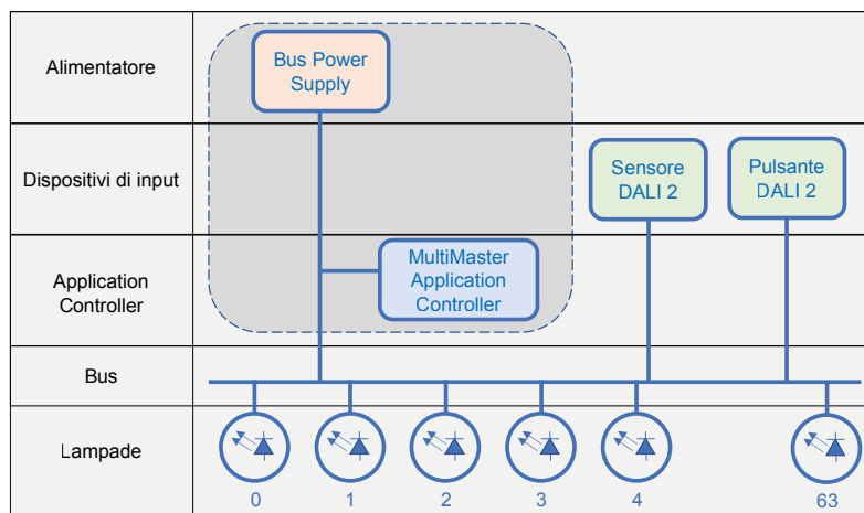
Figura 19. – Architettura DALI2
