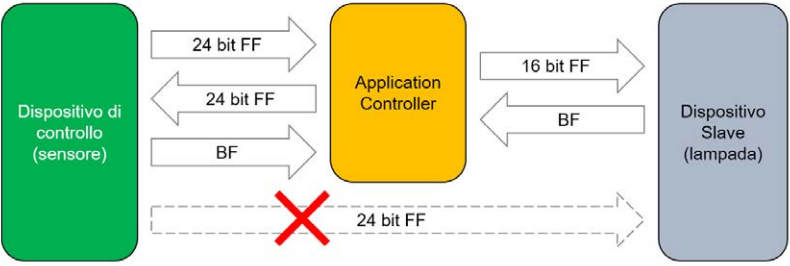
Figura 20. – Flusso dei messaggi in un sistema DALI 2
