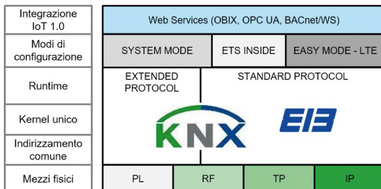
Figura 12. – Caratteristiche della tecnologia KNX
