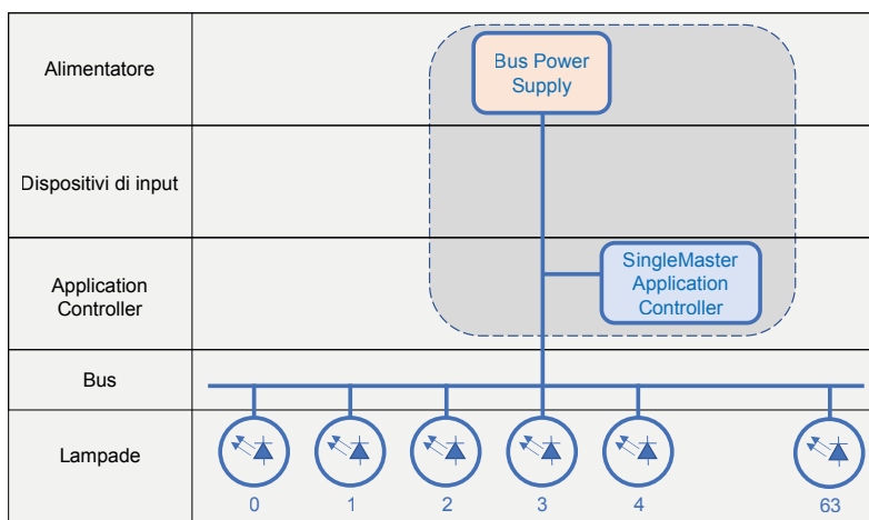
Figura 18. – Architettura DALI tradizionale
