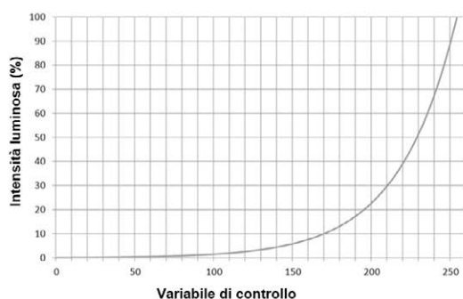
Figura 22. – Curva di dimming Logaritmica
