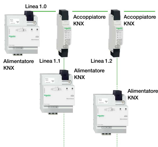
Figura 47. – Architettura con dorsale e linee bus TP
