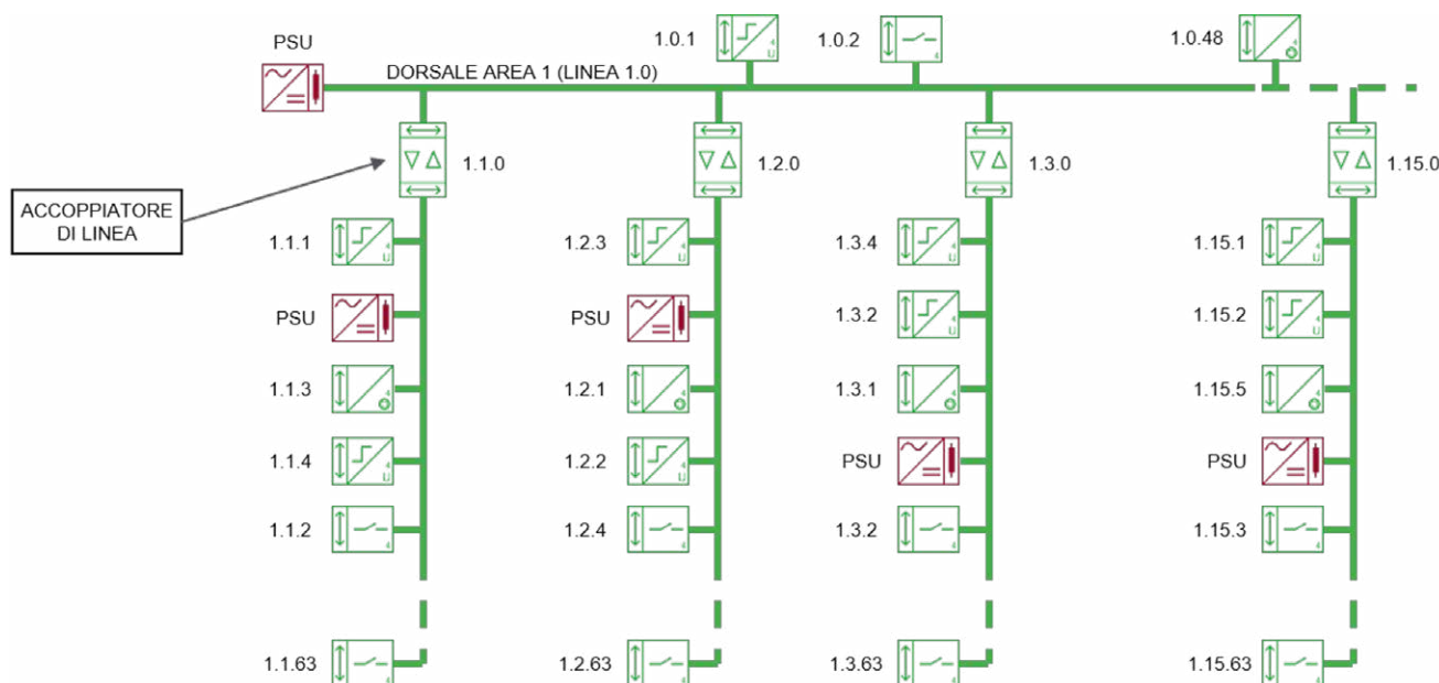
Figura 14. – Area KNX
