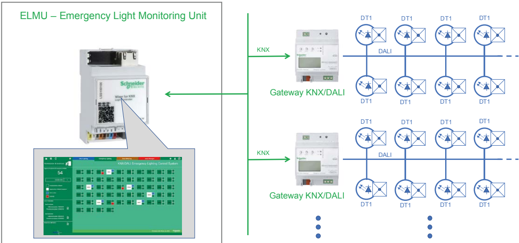
Figura 53. – Esempio di architettura di controllo di DALI Emergency Lighting tramite una supervisione KNX.
