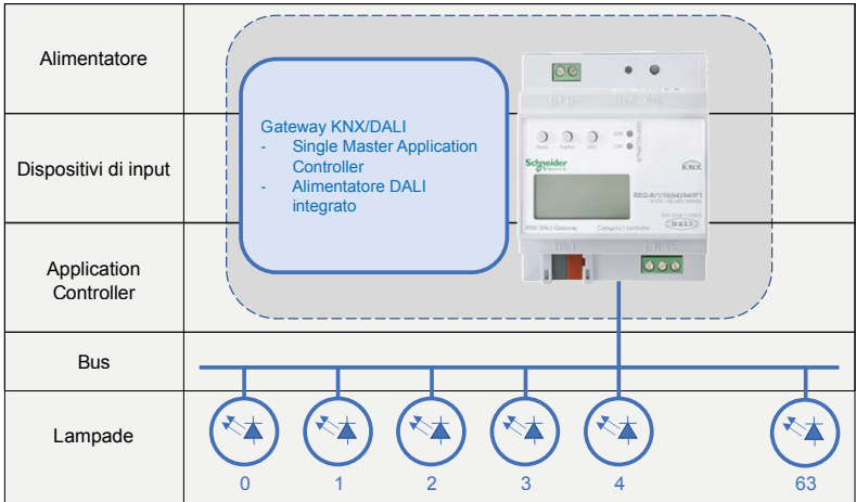
Figura 28. – Architettura DALI in un sistema KNX/DALI
