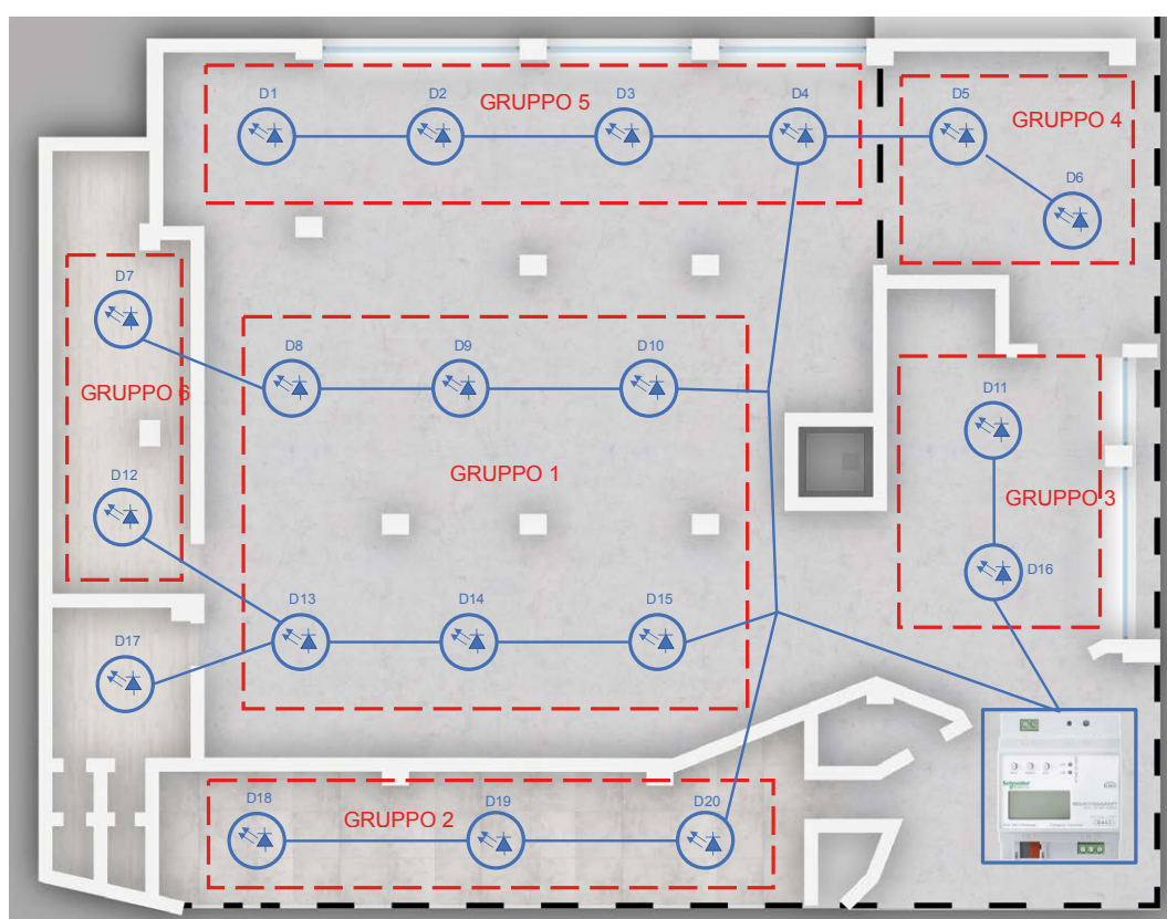
Figura 21. – Architettura DALI con divisione in gruppi
