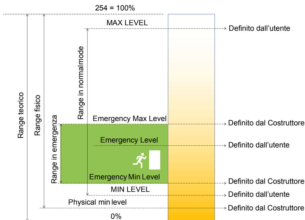
Figura 52. Livelli di flusso luminoso nelle lampade DALI DT1
