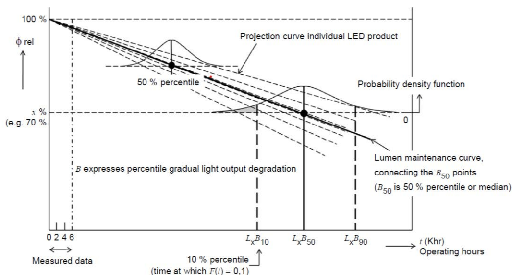
Figura 10. – Determinazione della vita utile delle sorgenti LED (EN 62717)
