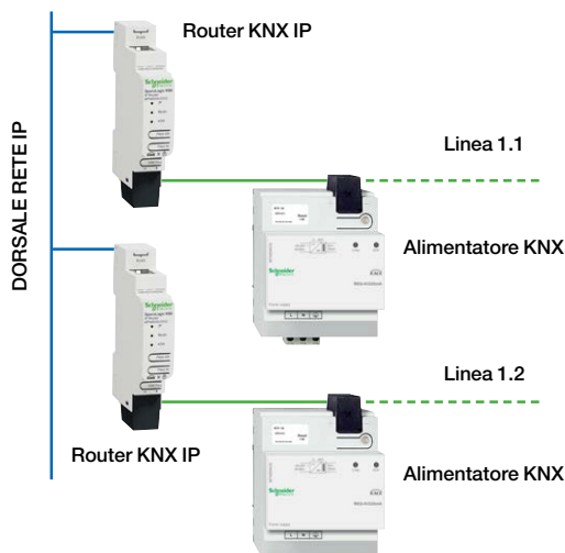
Figura 48. – Architettura con dorsale LAN e linee bus TP
