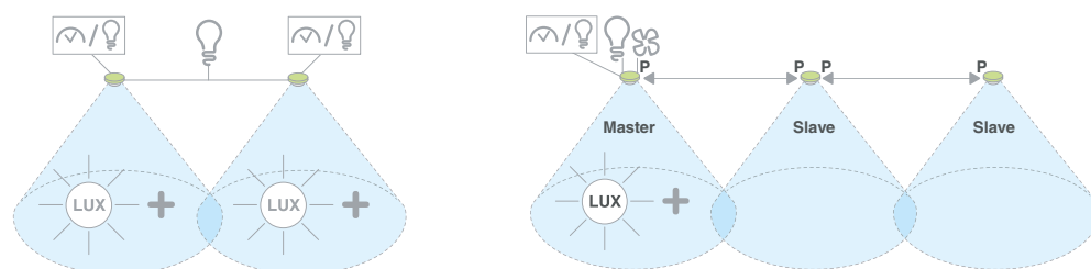
Figura 41. – Comportamenti diversi dei sensori presenza e controllo costante della luminosità
