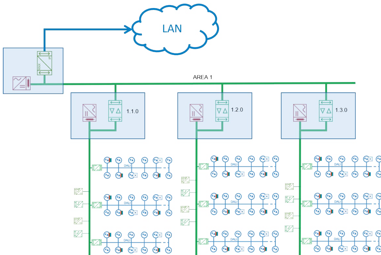
Figura 46. – Sistema LCS basato su 3 Linee KNX
