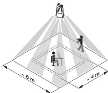
Figura 11. — Esempio di area di rilevamento di un sensore presenza da soffitto
