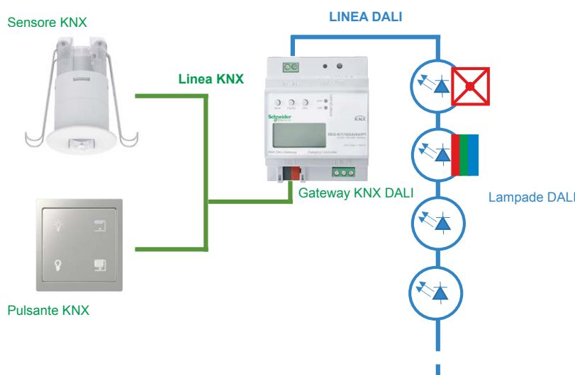
Figura 36. – Sensori KNX collegati ad una linea DALI tramite un gateway KNX DALI
