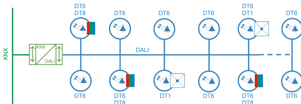
Figura 33. – Segmento DALI
