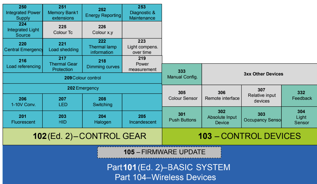
Figura 17. – Struttura dello Standard IEC 62386 (le parti in grigio devono ancora essere pubblicate)
