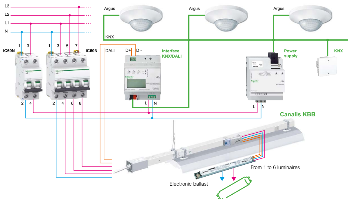
Figura 34. – Integrazione del Bus DALI nei condotti sbarra per illuminazione
