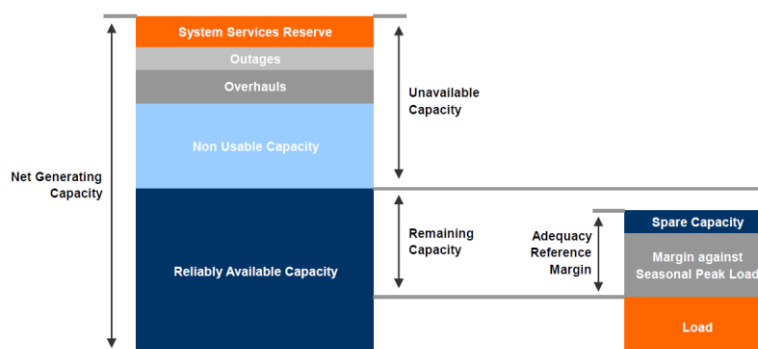
Grafico 3 – Schema della metodologia di calcolo dell'adequazione della generazione
