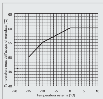
PUHZ-SW40/50
