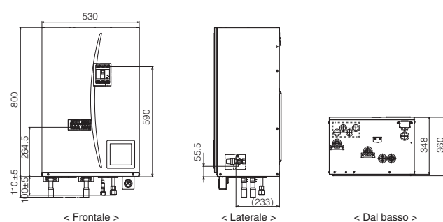
HYDROTANK EHST20C-VM6(S)B
