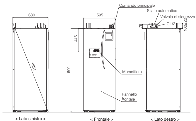
HYDROTANK EHST20C-VM6(S)B
