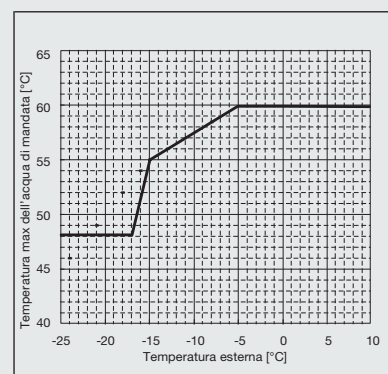
PUAZ-HW112YHA2 PUAZ-HW140YHA2
