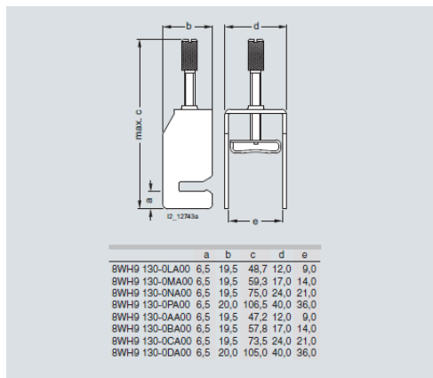
Morsetti schermati
