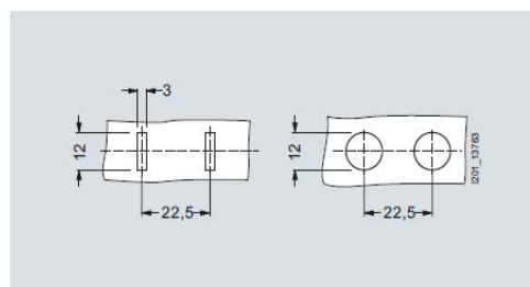
Taglio e dime foratura 8WH9 130-0CA00
