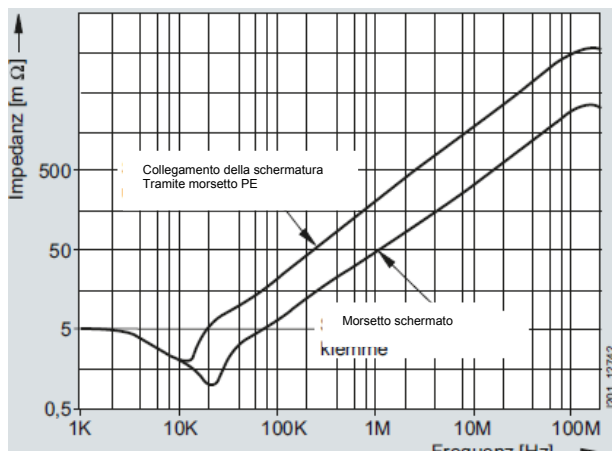
Confronto della schermatura tramite morsetto di terra PE rispetto al morsetto schermato
