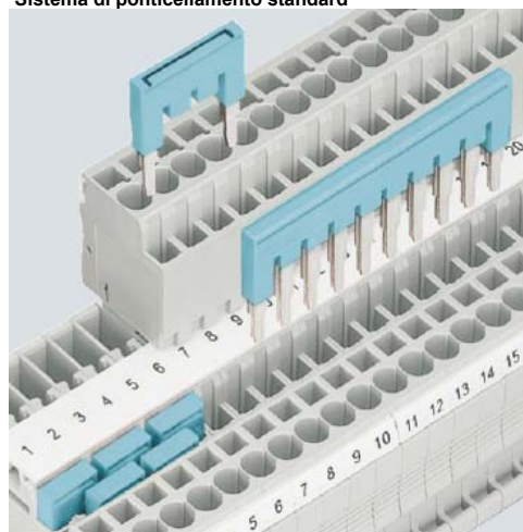
Sistema di ponticellamento standard
