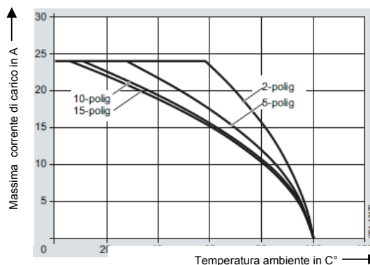
Curva di declassamento per 8WH5 004-0AF00
