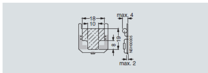
Vano per componenti elettronici
