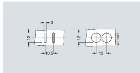
Morsetti schermati
