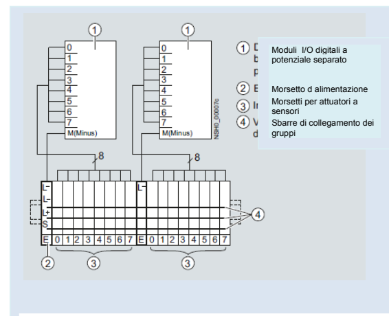
Morsetti per attuatori e sensori con moduli I/O digitali a potenziale separato
