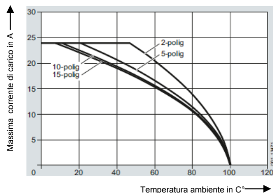
Curva di declassamento per 8WH5 000-0AF00
