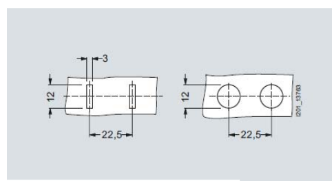
Taglio e dime foratura 8WH9 130-0DA00
