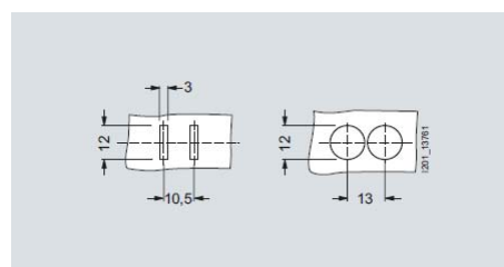
Taglio e dime foratura 8WH9 130-0AA00
