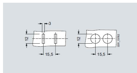
Taglio e dime foratura 8WH9 130-0BA00
