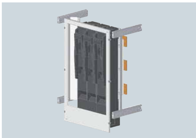
Configurazione con ingresso cavi dal basso
