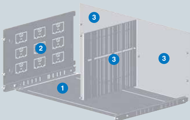
Segregazione per struttura profondità 600 mm e 800 mm
