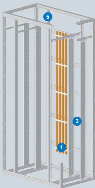
Sistemi di sbarre compatti 8GF57 piane, fissati con traverse, posteriori
