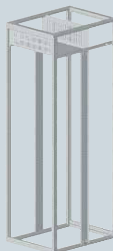
Sistema di sbarre principali in posizione standard superiore frontale o posteriore P = 800 mm
