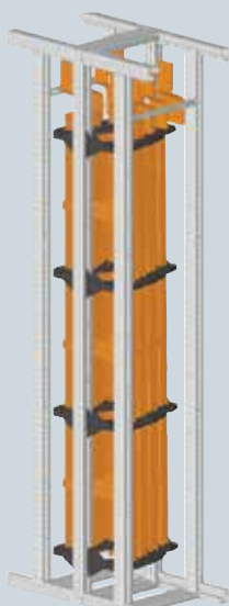
Sistema sbarre di distribuzione a gradini con sbarre profilate. Disposizione doppia affiancate
