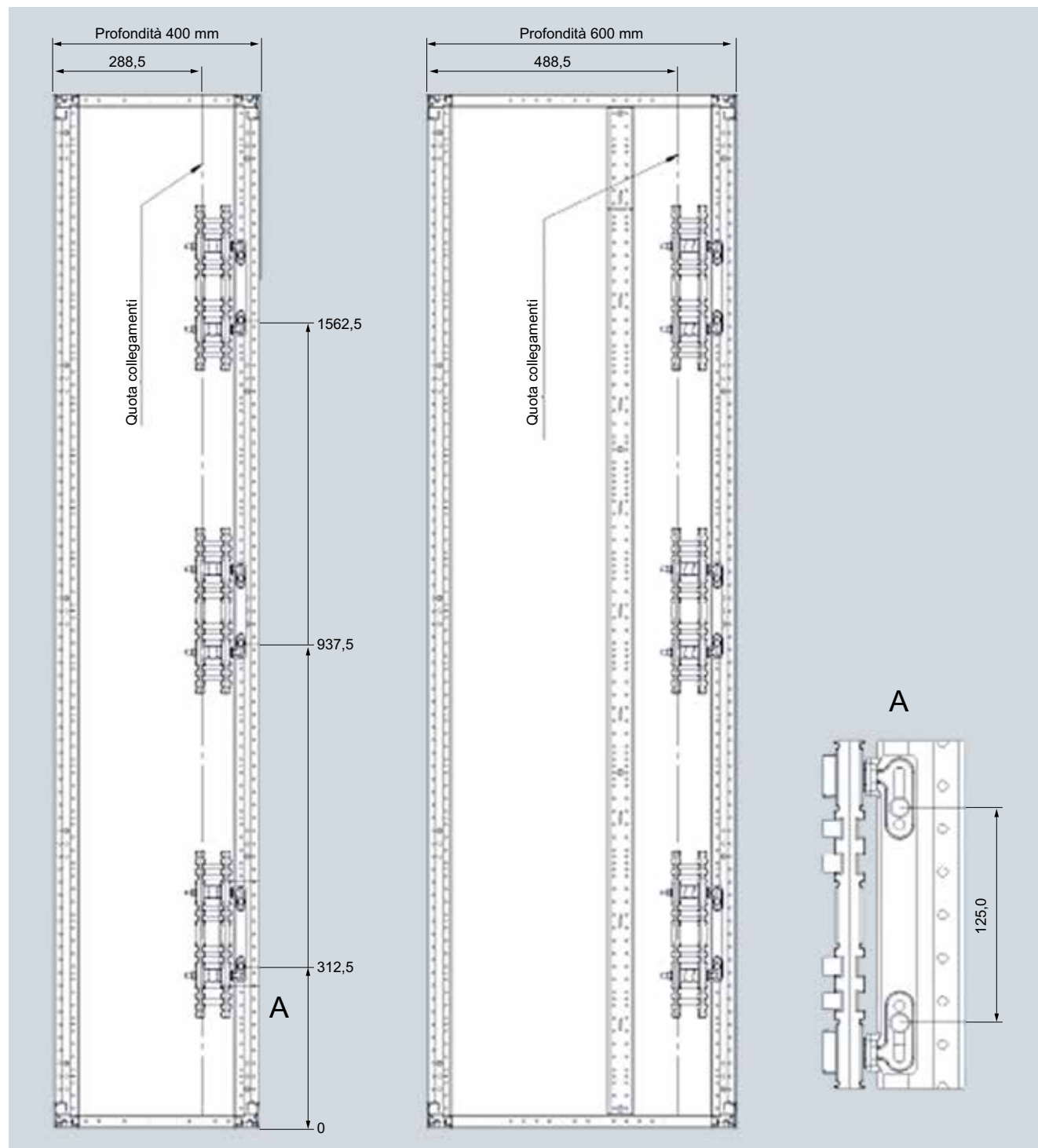
Vista in sezione struttura con 3 sistemi di sbarre
