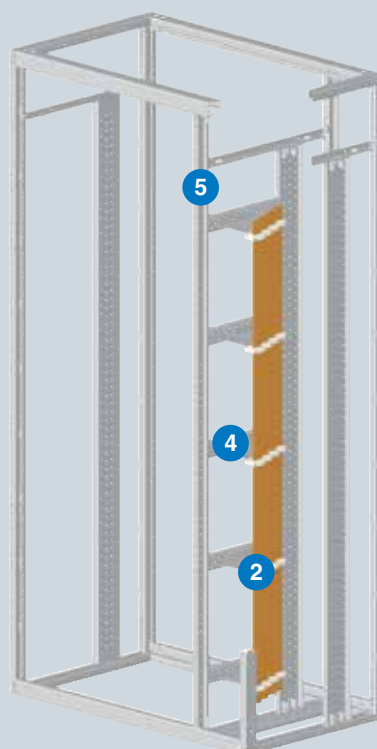
Sistemi di sbarre compatti 8GF57 a gradino, fissati con traverse, laterali
