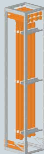
Sistema sbarre di distribuzione piane con sbarre rettangolari. Disposizione singola
