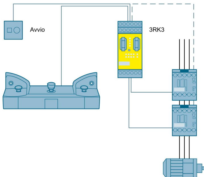
Figura 14-4 Comando a due mani fino a SIL 3 o PL e con un sistema di sicurezza modulare
