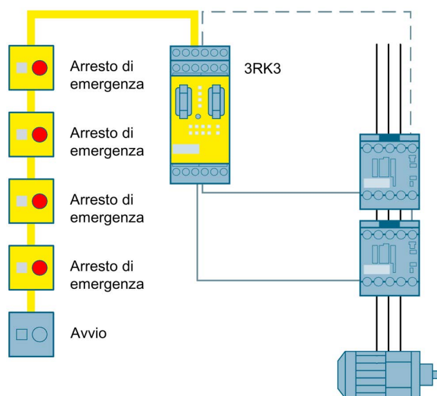
Figura 14-2 Disinserimento di arresto di emergenza tramite AS-i fino a SIL 3 o PL e con un sistema di sicurezza modulare
