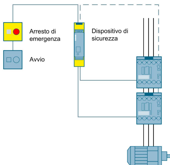
Figura 14-1 Disinserimento di arresto di emergenza fino a SIL 3 o PL e con un dispositivo di sicurezza
