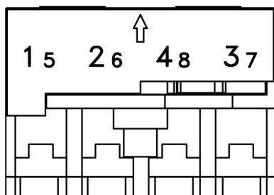
Figura 4-2 Indicazione delle posizioni d'inserzione sul supporto 4x
