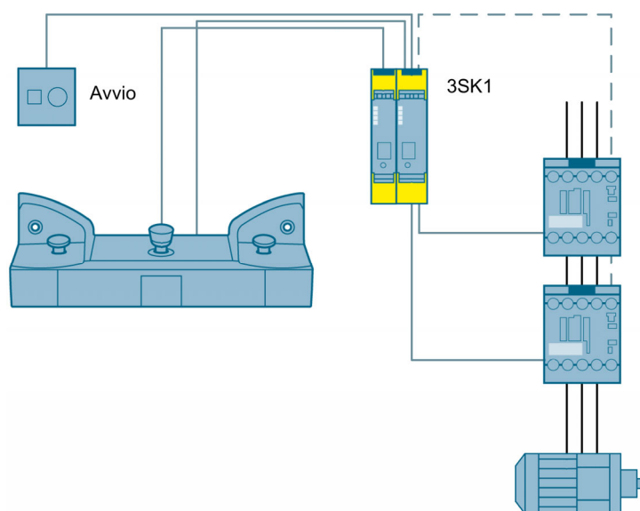
Figura 14-3 Comando a due mani fino a SIL 3 o PL e con un dispositivo di sicurezza
