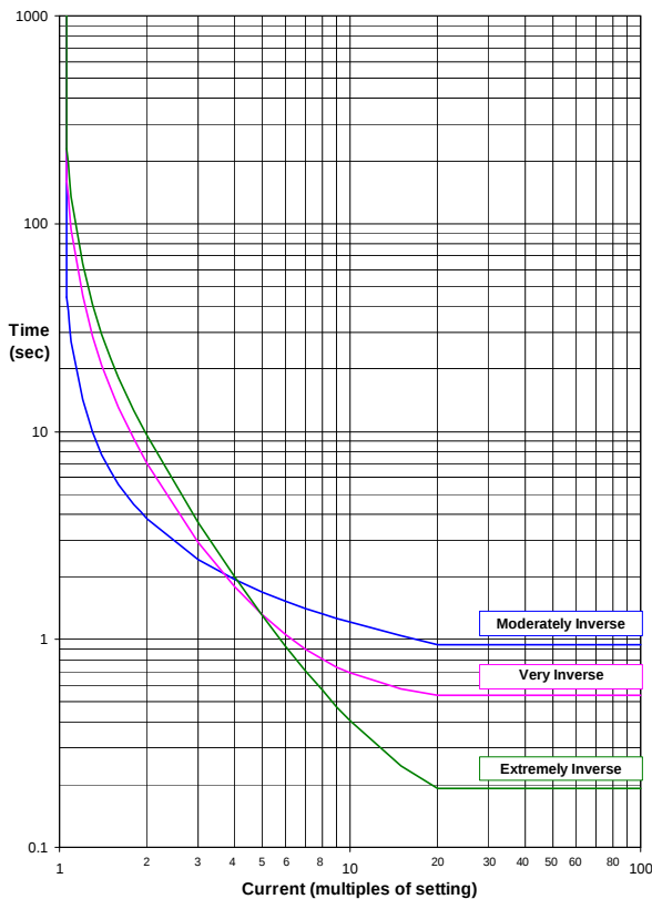
Fig 3. Curve ANSI di Massima Corrente
