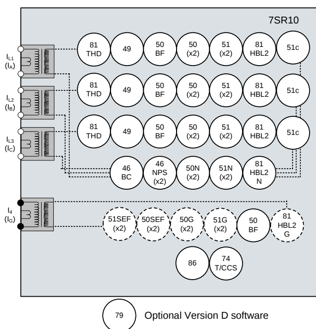
Fig 1. Relè di Massima Corrente Trifase+Terra
