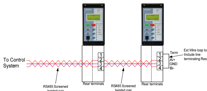
Fig 4. Tipica Connessione Tramite Porta RS485
