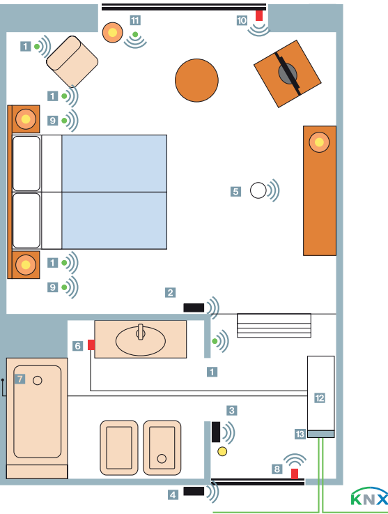
Controllo e automazione di una camera tipo Soluzione wireless
