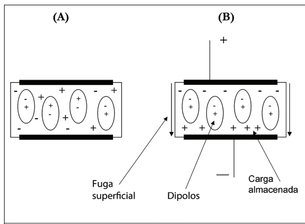
Figura 1: Alineación de moléculas polarizadas
