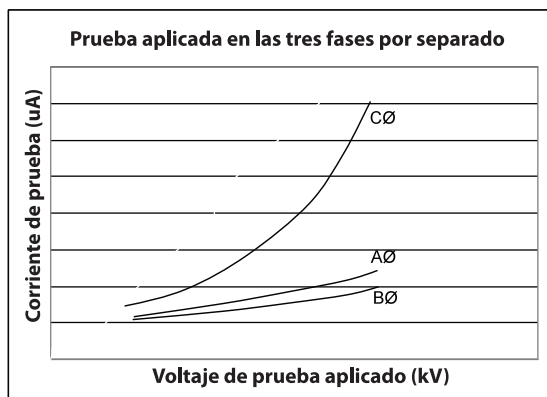
Figura 27: Prueba aplicada en las tres fases por separado
