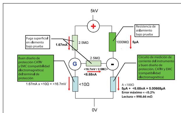
Figura 16: Circuito de medición con un terminal de protección de gran exactitud y baja impedancia
