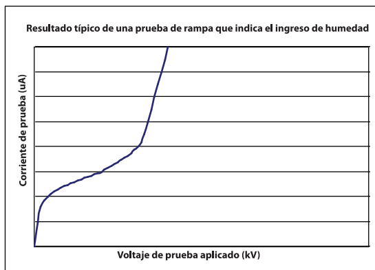
Figura 24: Resultado típico de una prueba de rampa que indica el ingreso de humedad
