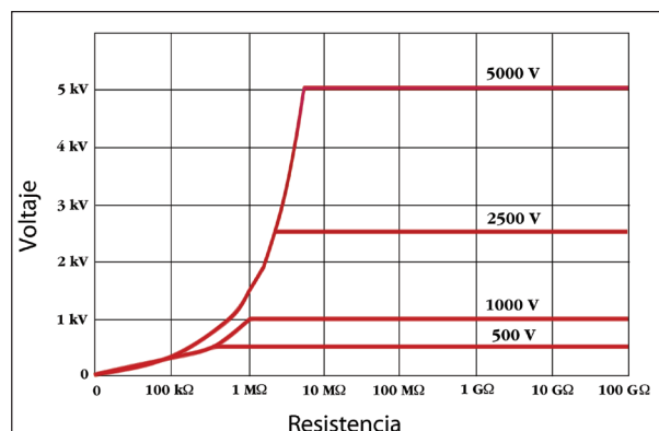
Figura 9: Buena curva de carga
