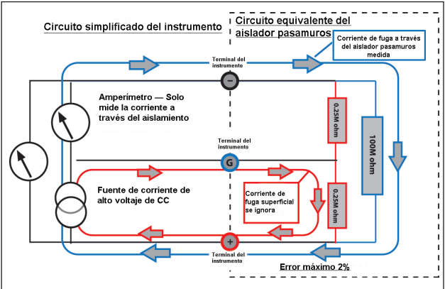
Figura 14: Circuito simplificado del instrumento
