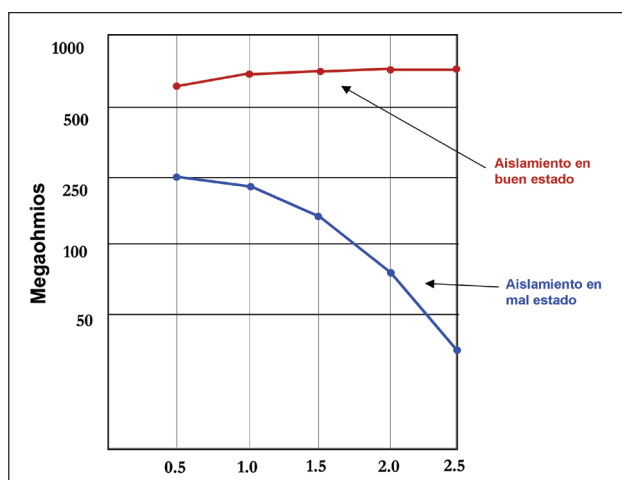
Figura 21: Gráfico de escalón de voltaje
