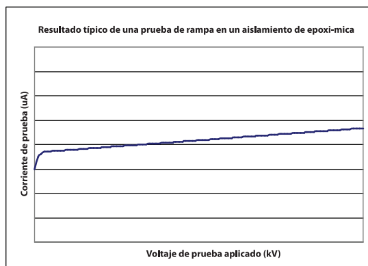
Figura 22: Resultado típico de una prueba de rampa en un aislamiento de epoxi-mica
