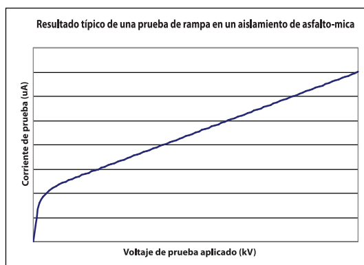
Figura 23: Resultado típico de una prueba de rampa en un aislamiento de asfalto-mica
