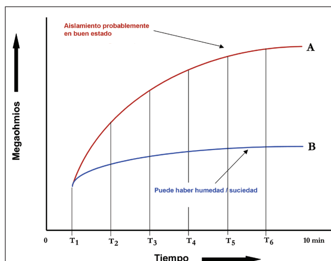
Figura 19: Gráfica de prueba de tiempo-resistencia
