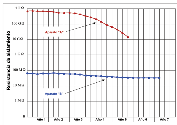
Figura 18: Comparación de tendencias de los resultados de las pruebas
