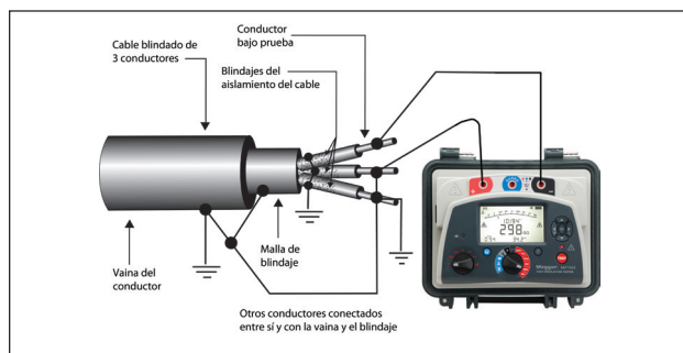
Figura 4: Conexión a un cable de potencia blindado
