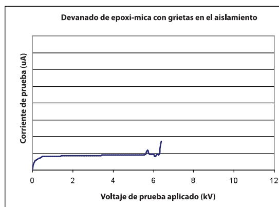
Figura 26: Devanado de epoxi-mica con grietas en el aislamiento
