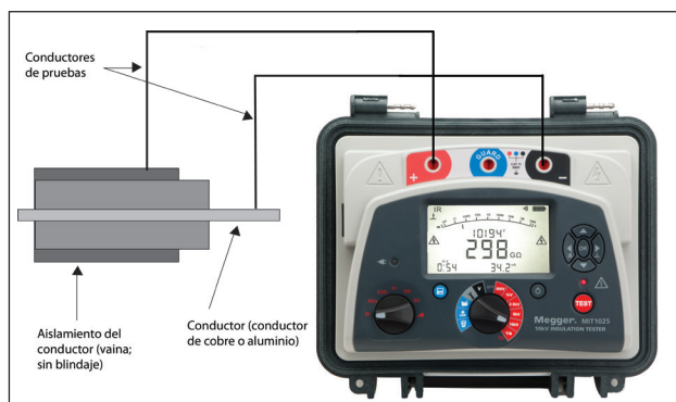
Figura 3: Conexión simplificada a un cable
