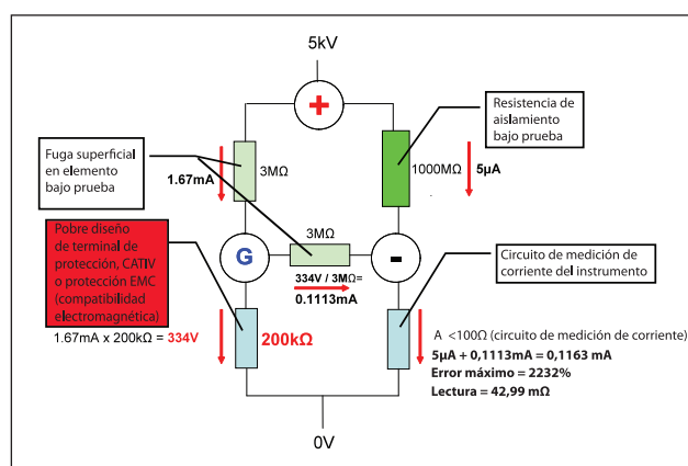
Figura 15: Circuito de medición "protegido" por una protección de alta impedancia
