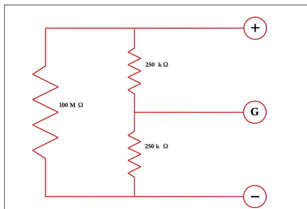
Figura 12: Diagrama de terminal de protección
