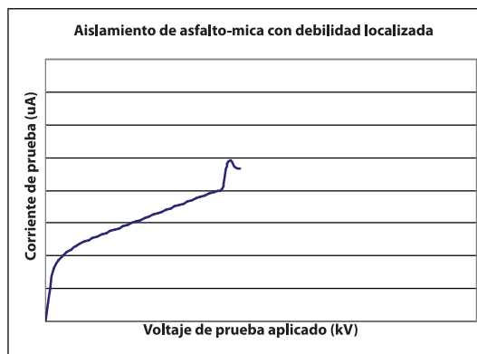
Figura 25: Aislamiento de asfalto-mica con debilidad localizada
