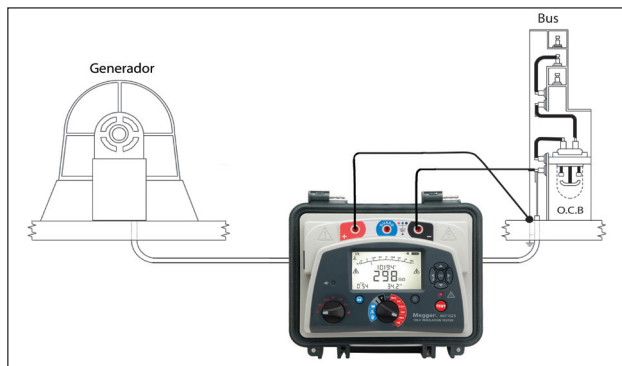
Figura 7: Conexión a un generador de CA
