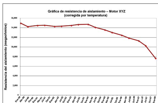
Figura 33: Gráfica de resistencia de aislamiento corregida por temperatura
