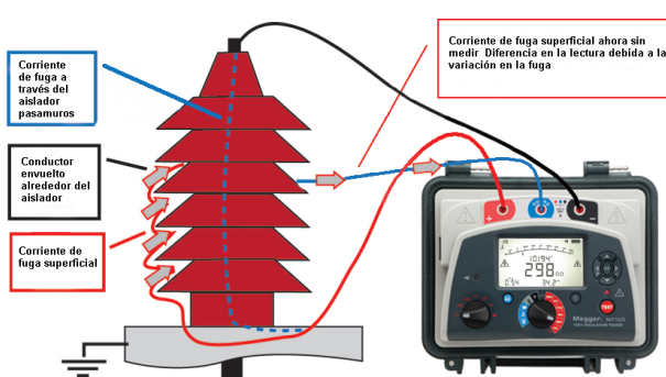
Figura 13: Ejemplo con un aislador pasamuros de alto voltaje
