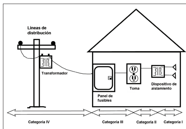
Figura 31: Alimentación eléctrica separada en categorías
