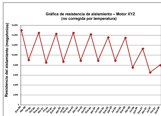
Figura 32: Gráfica de resistencia de aislamiento no corregida por temperatura
