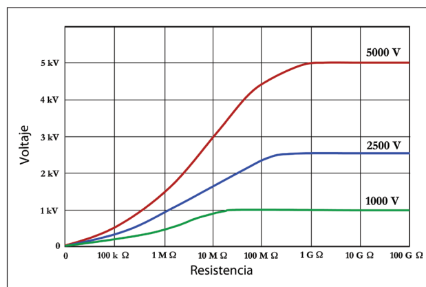
Figura 10: Pobre curva de carga
