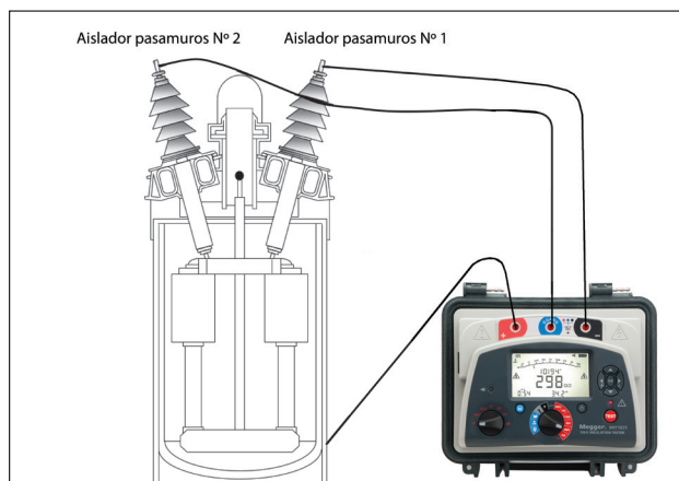
Figura 5: Conexión a un interruptor de circuito
