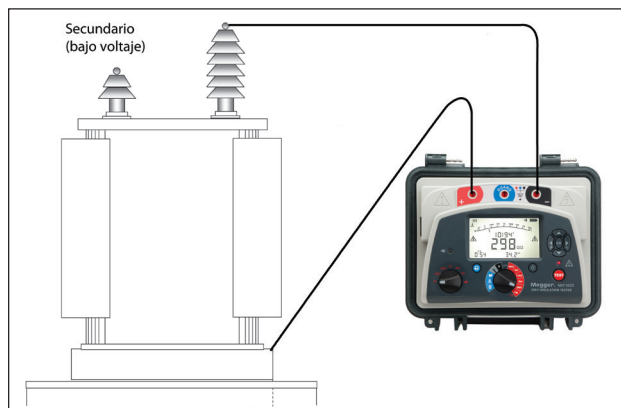
Figura 6: Conexión a un transformador de potencia
