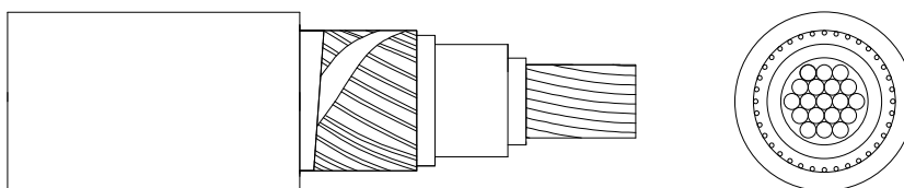
X-VOLT® RHZ1 6/10 kV
