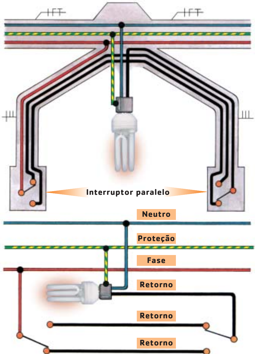
Esquema equivalente
