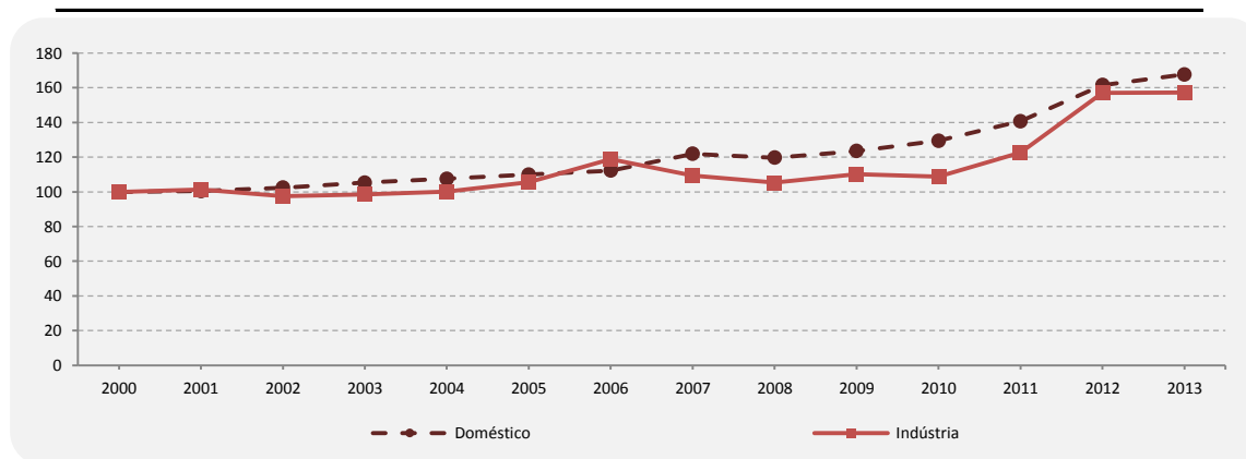
Figura 61 - Evolução dos preços médios com taxas da Eletricidade ao consumidor final em Portugal por setor (2000=100)
