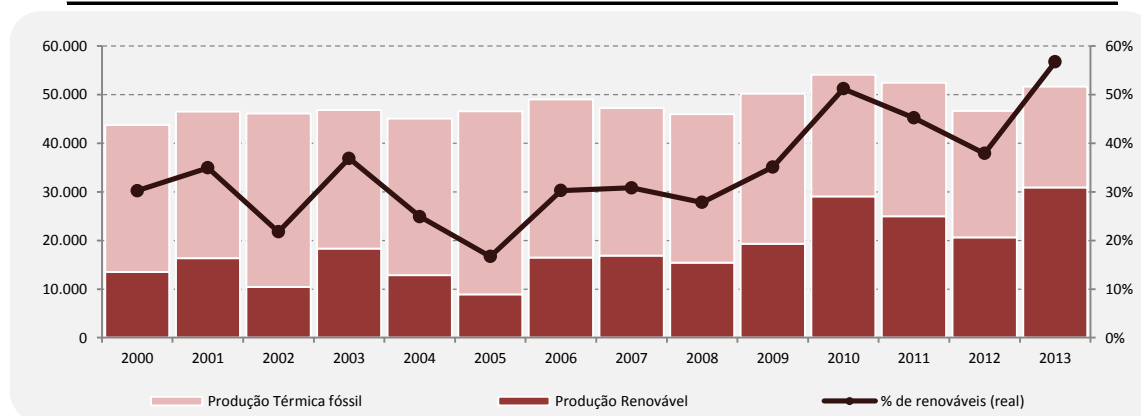
Figura 54 - Evolução da produção bruta de eletricidade em Portugal por tipo de fonte (GWh)
