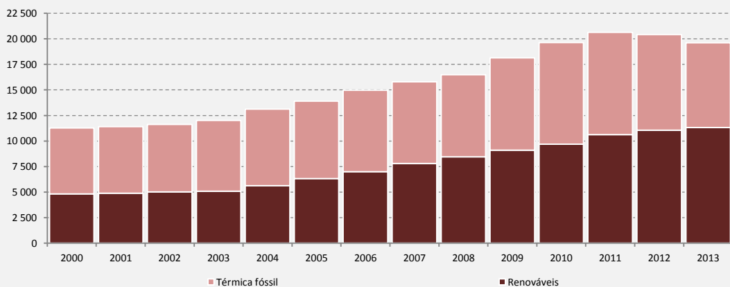
Figura 57 - Evolução do mix de capacidade instalada para produção de eletricidade em Portugal (MW)
