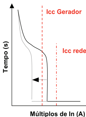
Figura 7 · Regulação do magnético nas curvas.
