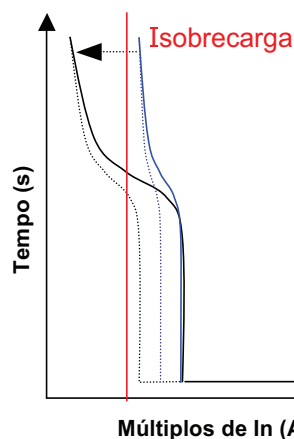
Figura 5 · Regulação do térmico nas curvas.
