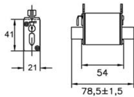
Size 000
