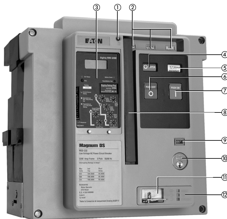
Magnum DS Drawout Breaker
