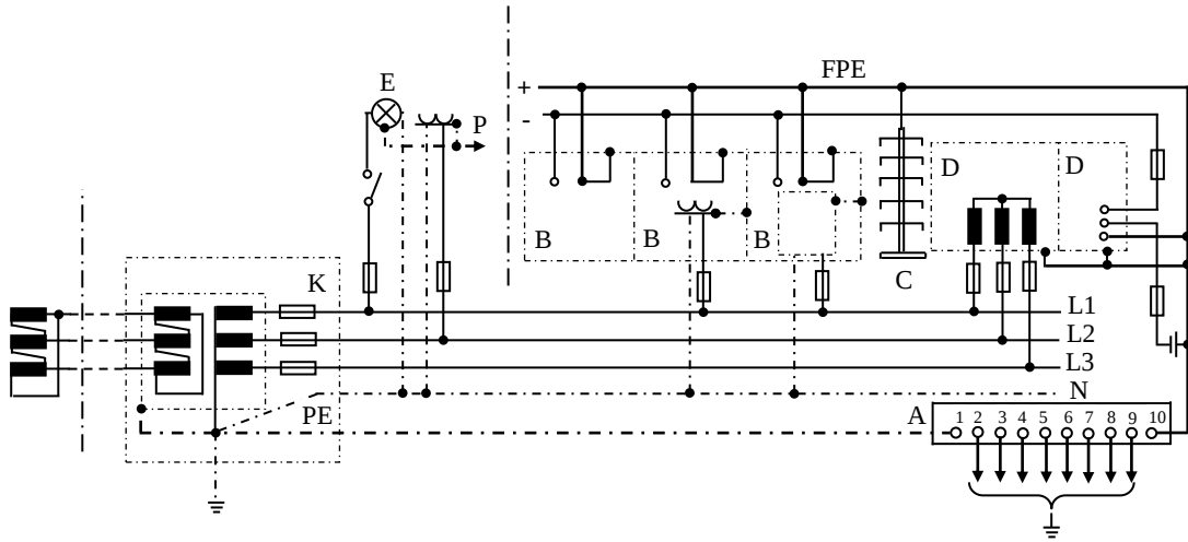
Şekil-16 Madde 21-b1'de belirtilen bir iletişim sisteminin fonksiyon ve koruma topraklamasına örnek (Not: Bu şekil mecburi olmayıp, yalnızca bir fikir vermek amacıyla taşınmaktadır.)
