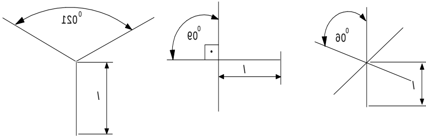
Şekil-T.8 Yıldız topraklayıcı çeşitleri
