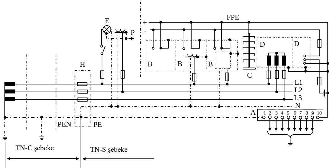
Şekil-17 Madde 21-b2'de belirtilen bir iletişim tesisinin fonksiyon ve koruma topraklamasına örnek (Not: Bu şekil mecburi olmayıp, yalnızca bir fikir vermek amacıyla taşımaktadır.)
