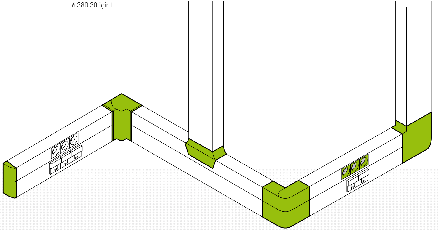
Değişken iç köşeler 80°/120°
