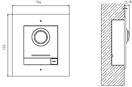
1 Modül Sıva Altı Montaj
