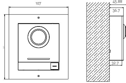
1 Modül Sıva Üstü Montaj
