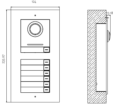
2 Modül Sıva Altı Montaj
