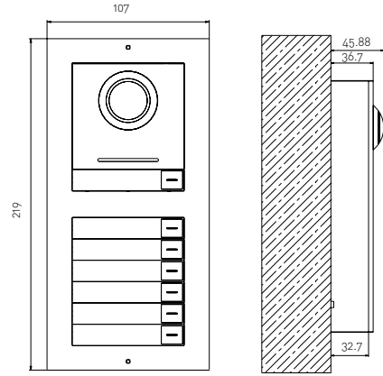
2 Modül Sıva Üstü Montaj
