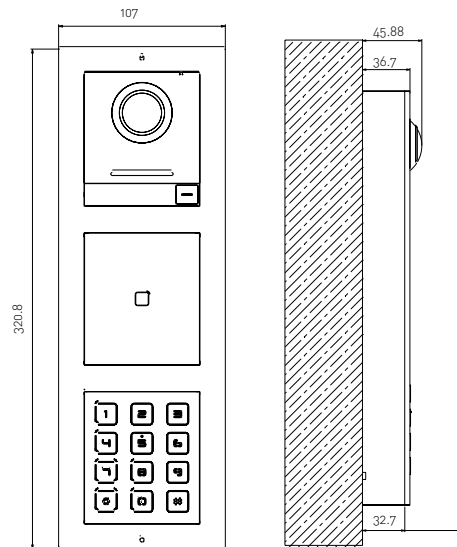
3 Modül Sıva Üstü Montaj
