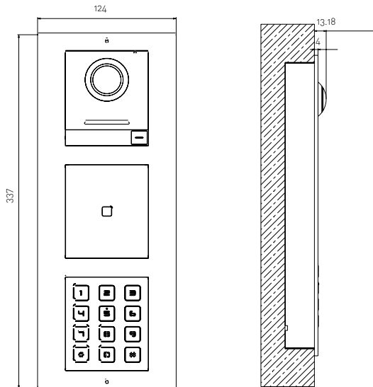
3 Modül Sıva Altı Montaj
