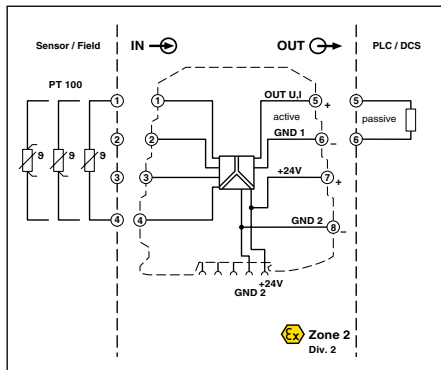
MINI MCR-SL-PT 100-UI-NC için bağlantı şekli
