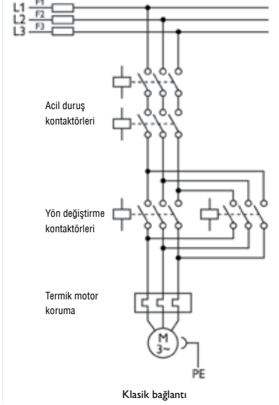
Klasik bağlantı
