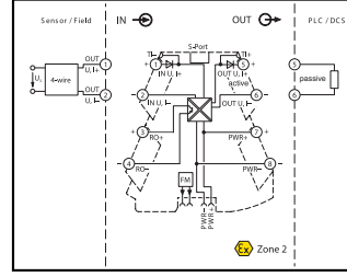
MINI MCR-2-UNI-UI-UIRO-PT için bağlantı şekli
