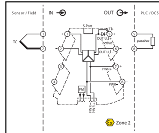
MINI MCR-2-TC-UI-PT için bağlantı şekli
