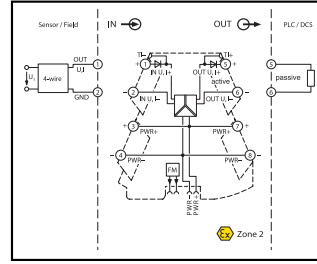
MINI MCR-2-UI-UI-PT için bağlantı şekli
