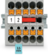
MPT klemensler, köprülenebilir, etiketlenebilir ve test edilebilir. MPT 1,5/S sadece 3.5 mm'dir.
