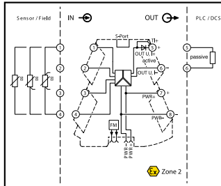
MINI MCR-2-RTD-UI-PT için bağlantı şekli
