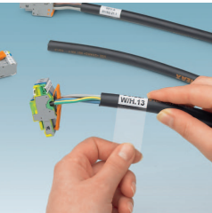
MM-WML..., WML..., US-WML... etiketler yazı alanı ve koruyucu şeffaf folyodan oluşur. Folyo yazının üzerine kapanarak kirlenme ve aşınmaya karşı koruma sağlar.
