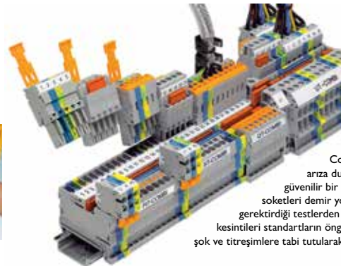
Combi fiş-soketli bağlantı sistemi ile hem sinyal hem de güç devreleri fiş-soketli olarak bağlanabilirler. Combi sistemiyle ray klemenslere bağlantının yanı sıra, panel geçişi yapılabilir ya da iki kablo havada bağlanabilir.
