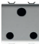
GW 14 298 2P+E-16 A-250 V ac
